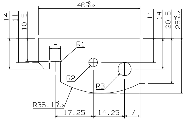
AH1 SERIAL 外形抜寸法図
