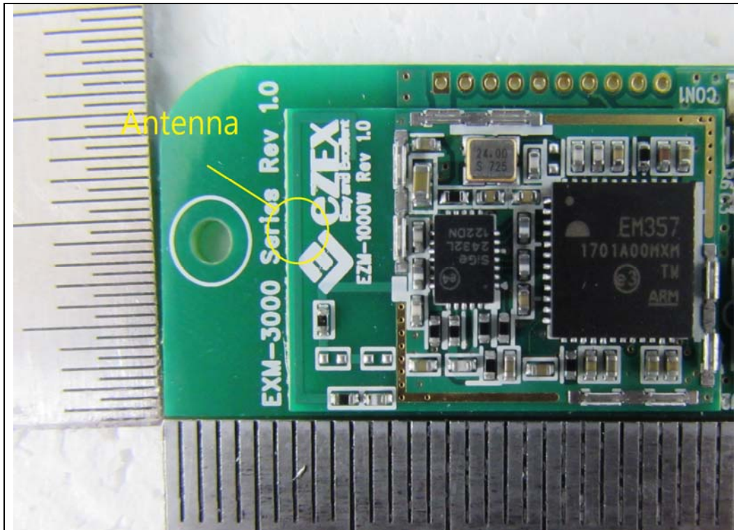
<Zigbee Antenna>
