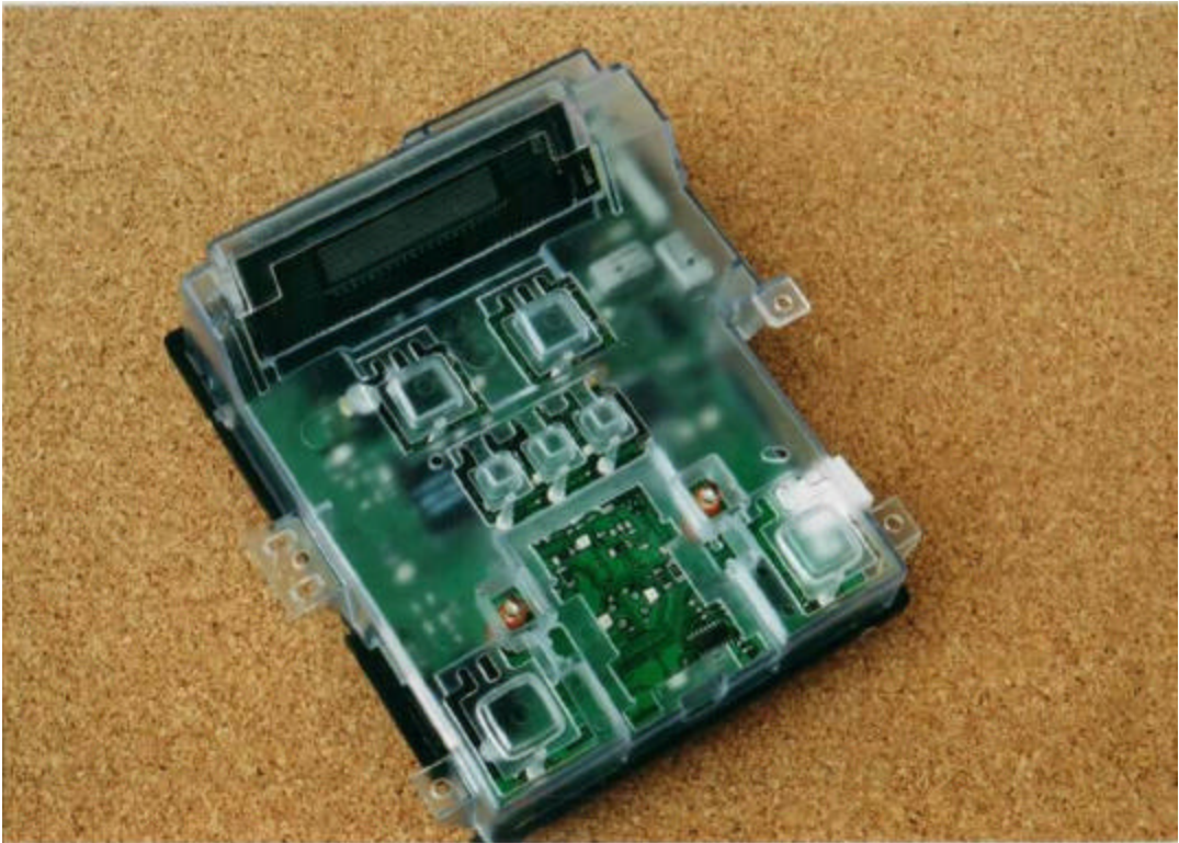
FN145-JB Top
