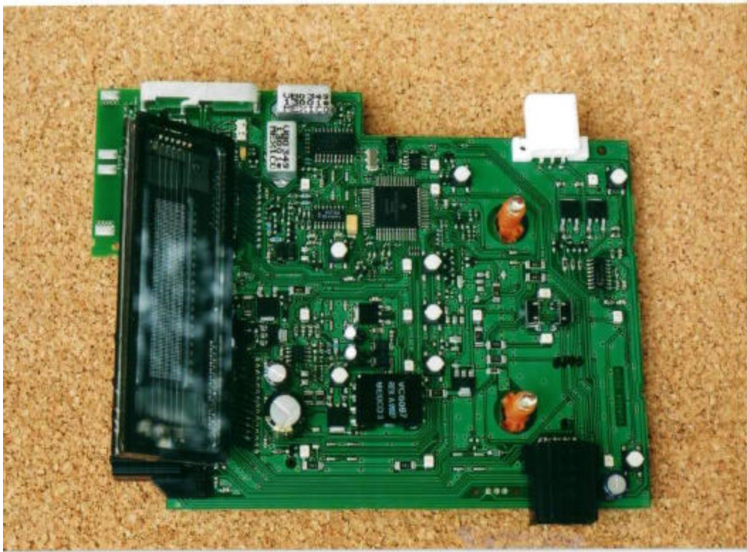
FN145-FB PCB - Top
