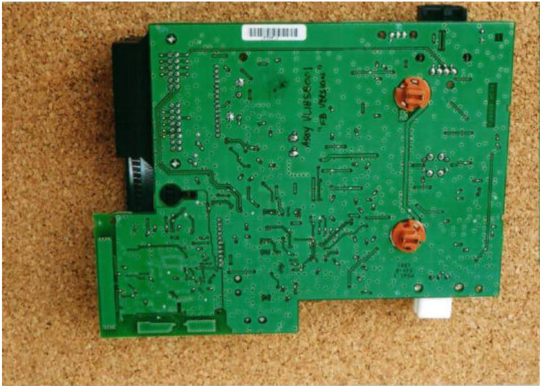
FN145-FB PCB - Bottom
