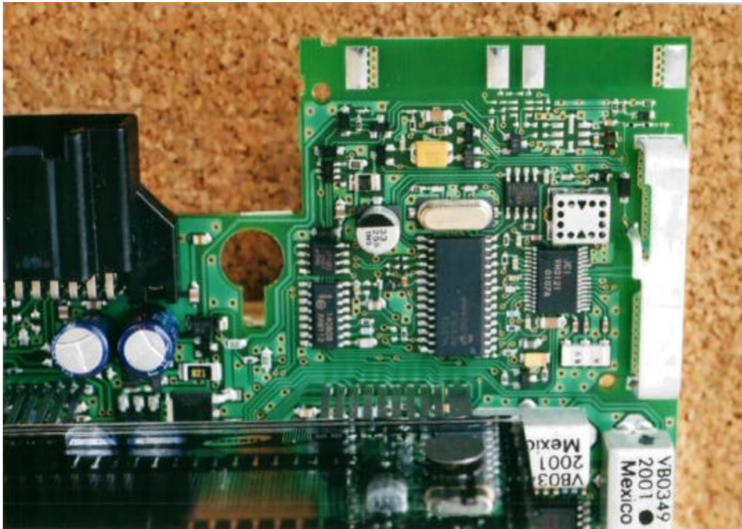
FN145-JB RF Section - Top
