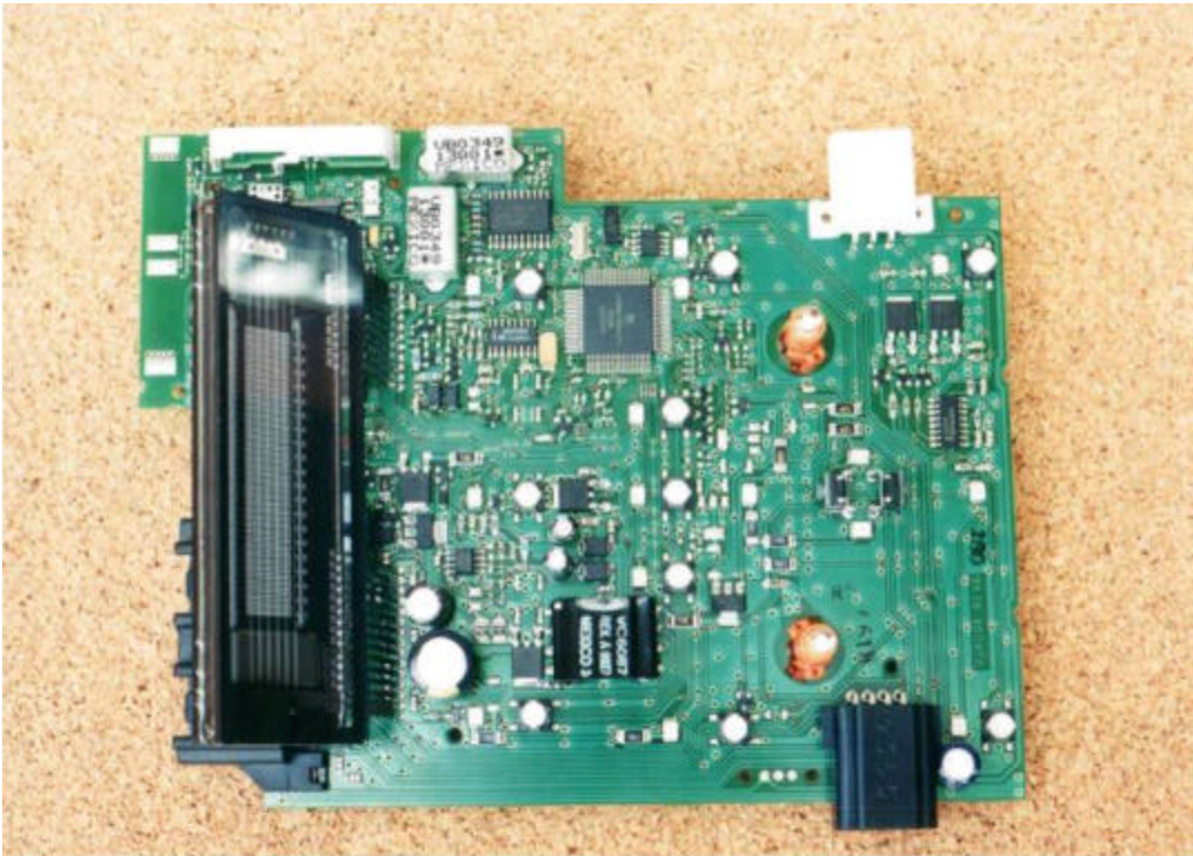
FN145-DB PCB - Top
