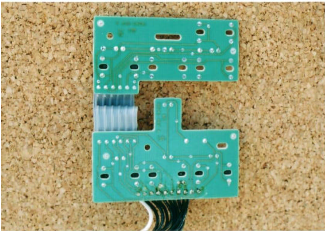
CPSIHL3 Keypad PCB - Top
