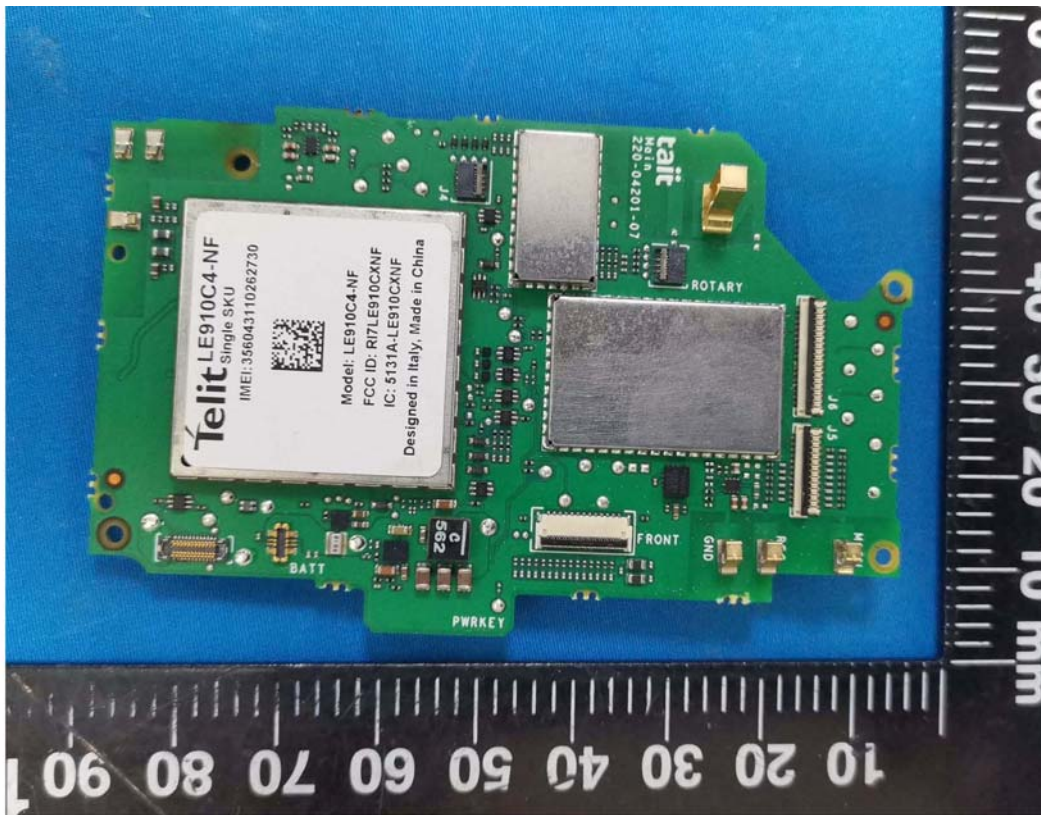
3G/4G Module
