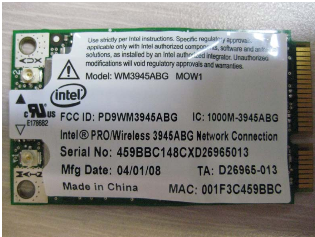
WLAN module
