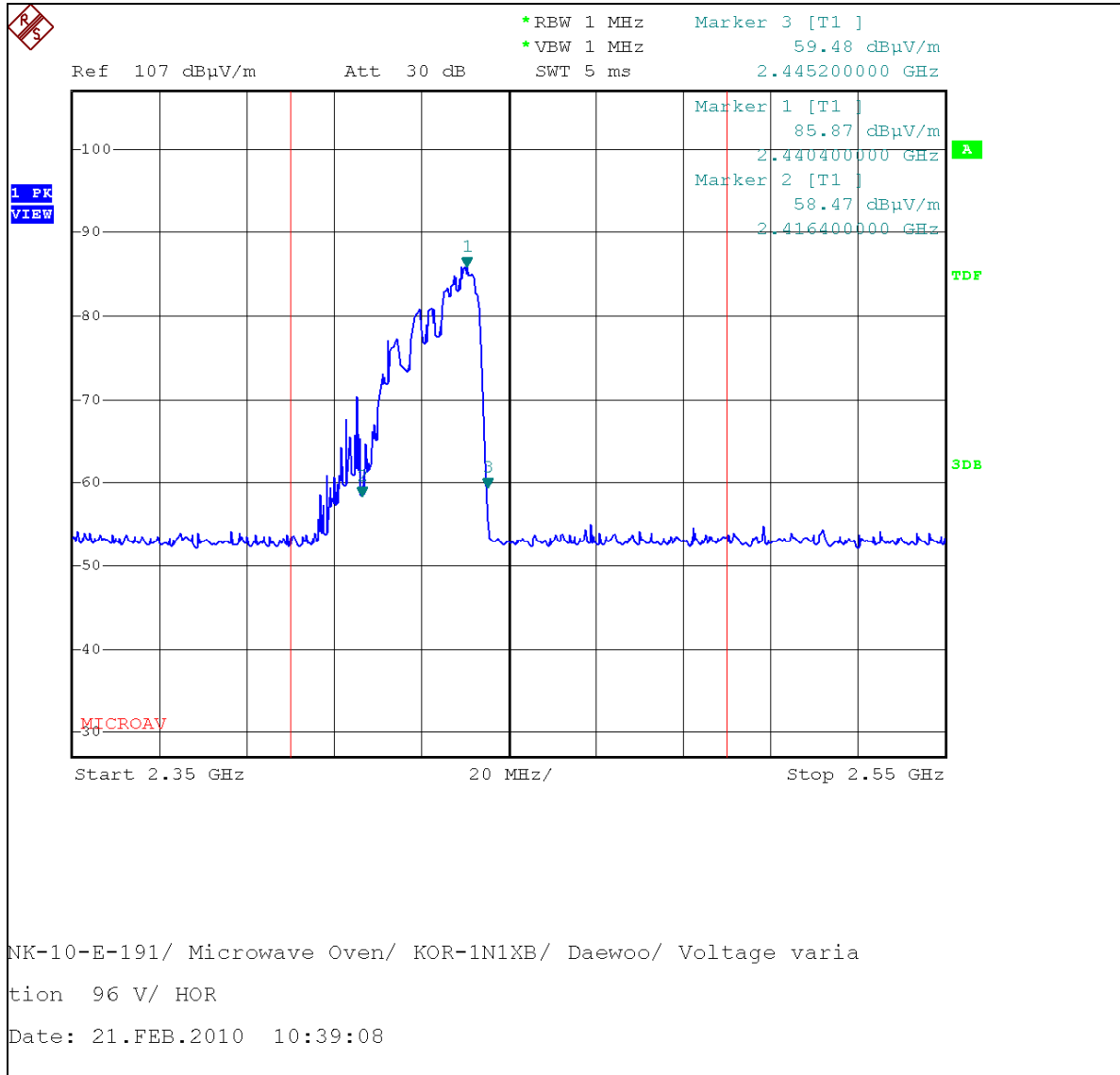
Magnetron : RM269_Horizontal (96 V, 1000 ml)
