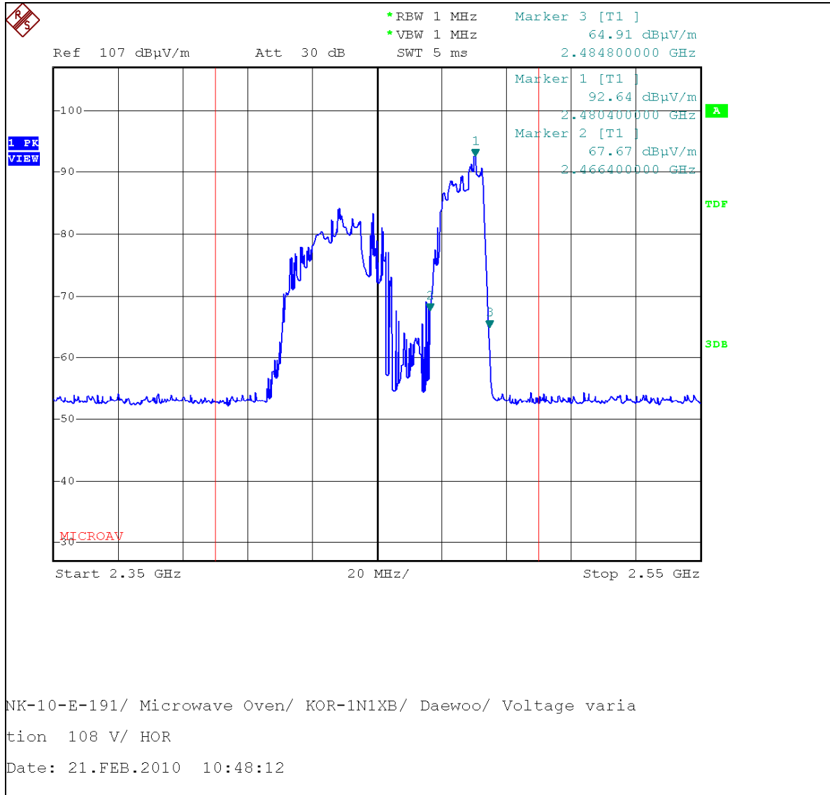
Magnetron : RM269_Horizontal (108 V, 1000 ml)
