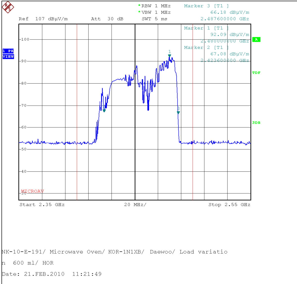
Magnetron : RM269_Horizontal (120 V, 600 ml)
