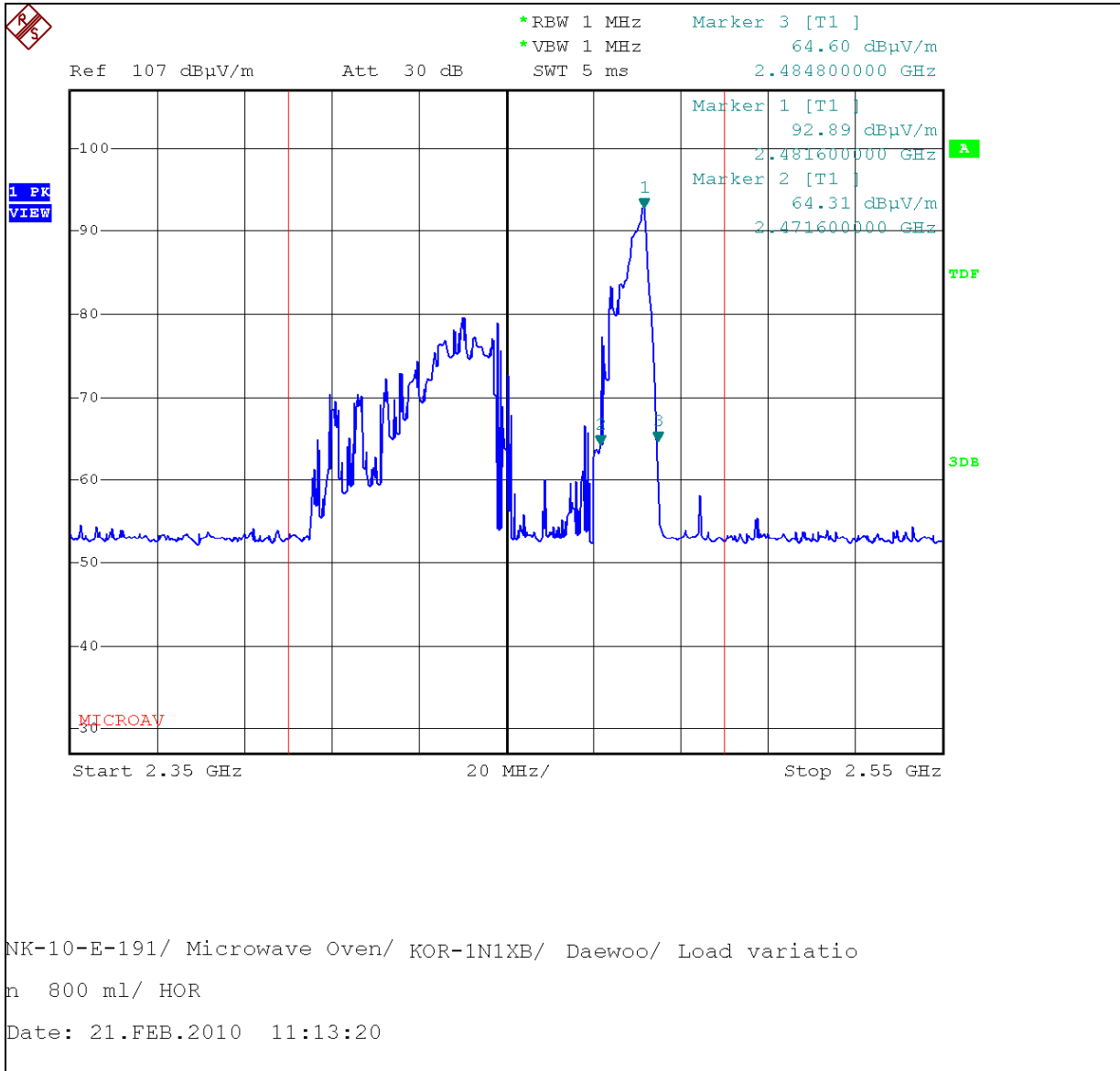
Magnetron : RM269_Horizontal (120 V, 800 ml)
