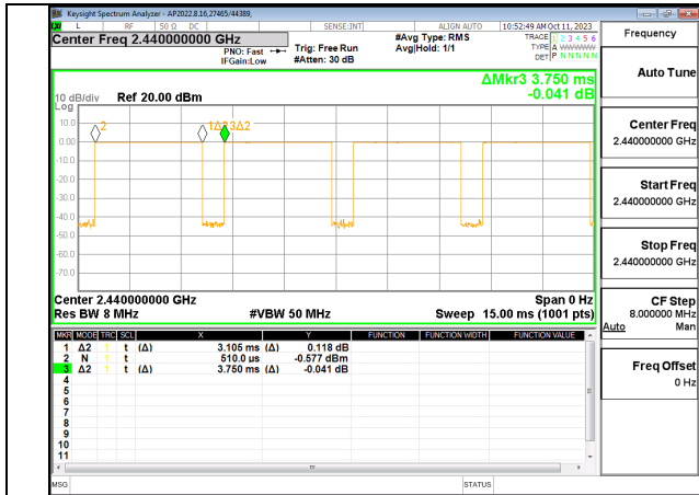
DUTY CYCLE BLE 125kbps
