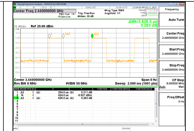
DUTY CYCLE BLE 2Mbps
