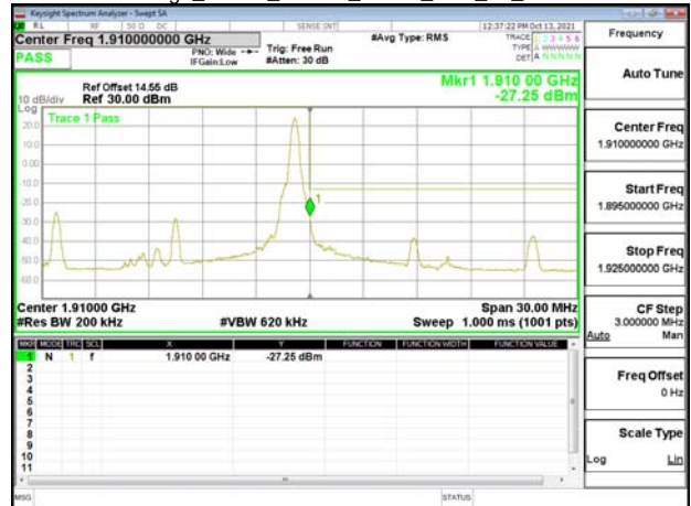
Band Edge_Band2_15MHz_OPSK_RB1_74_CH19125
