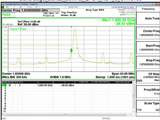
Band Edge_Band2_20MHz_OPSK_RB1_0_CH18700
