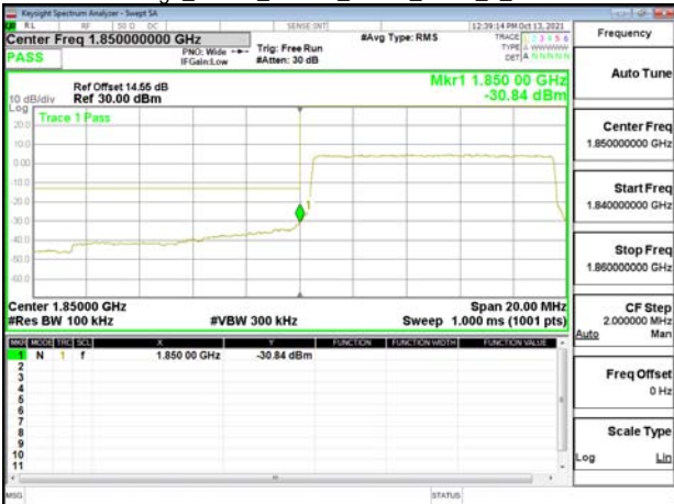
Band Edge_Band2_10MHz_OPSK_RB50_0_CH18650
