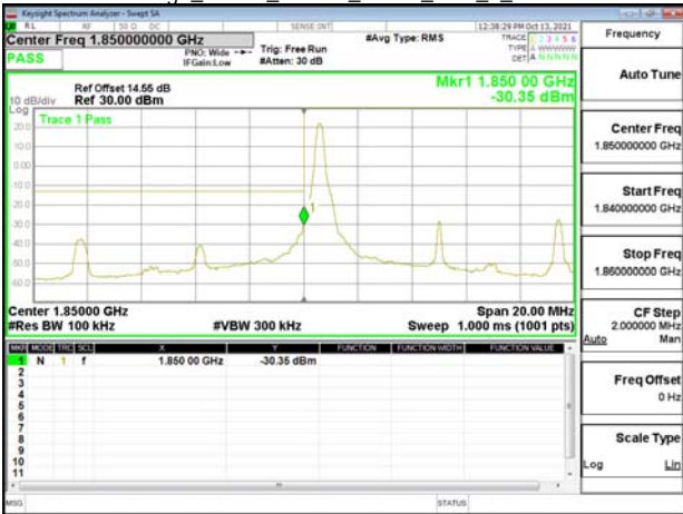
Band Edge_Band2_10MHz_OPSK_RB1_49_CH19150
