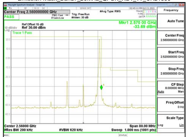
Emission Mask_Band7_20MHz_OPSK_RB1_99_CH21350
