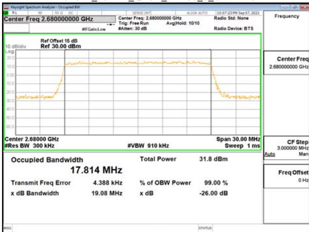
Band41_20MHz_QPSK_RB100_0_CH41490
