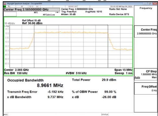
Band7_10MHz_QPSK_RB50_0_CH21400
