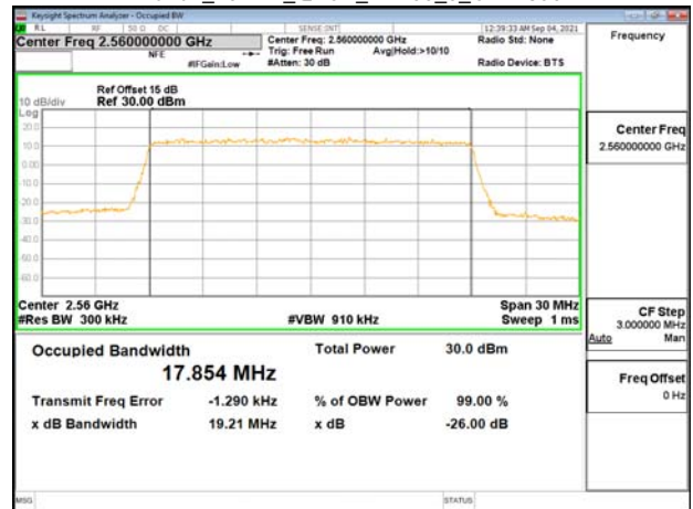
Band7_20MHz_QPSK_RB100_0_CH21350
