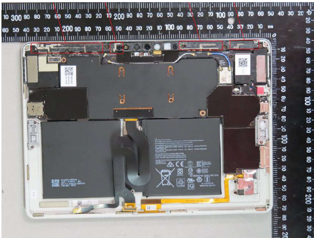
NFC Antenna
