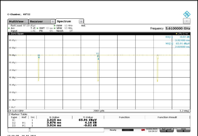
13:19:38 14.04.2021 802.11ax HE80 OFDMA, RU size 26T MODE
