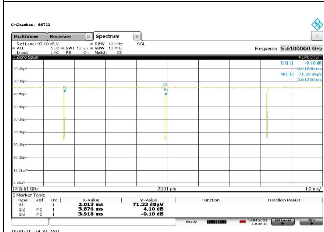
13:18:13 14.04.2021 802.11ax HE80 OFDMA, RU size 52T MODE
