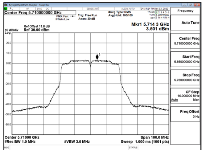
802.11n_40MHz_CHO_5710MHz_UNII 3
