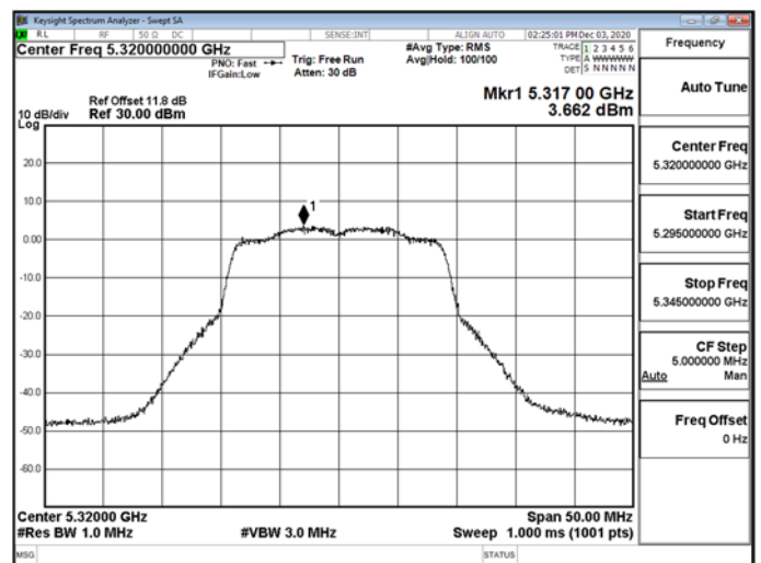
802.11n_20MHz_CH1_5320MHz-5320
