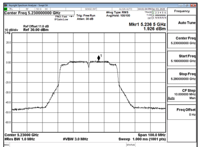
802.11n_40MHz_CH1_5230MHz-5230
