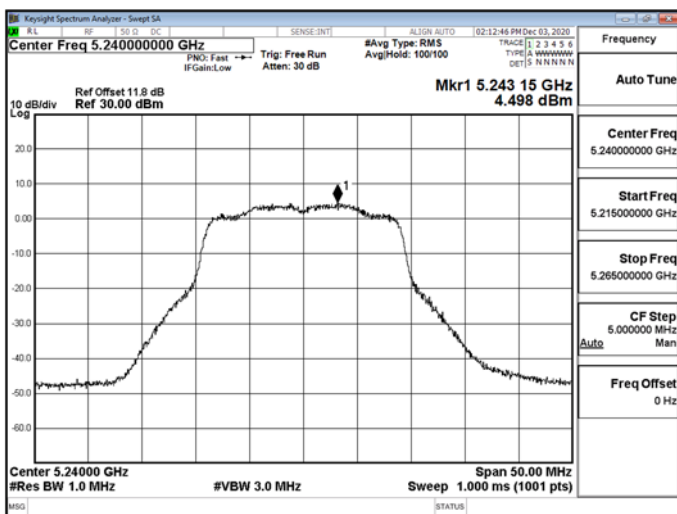
802.11n_20MHz_CH1_5240MHz-5240
