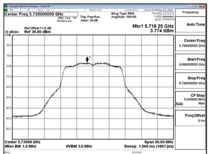
802.11n_20MHz_CHO_5720MHz_UNII 2C
