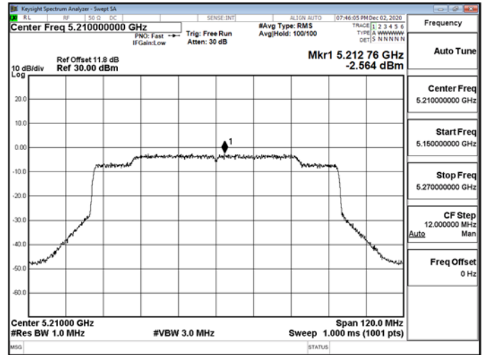
802.11ax_80MHz_RU_484_65_5210MHz-5210
