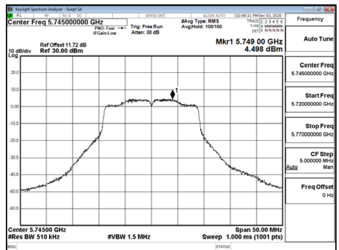
802.11n_20MHz_CH1_5745MHz-5745
