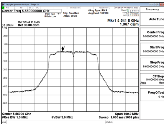
802.11n_40MHz_CHO_5550MHz-5550
