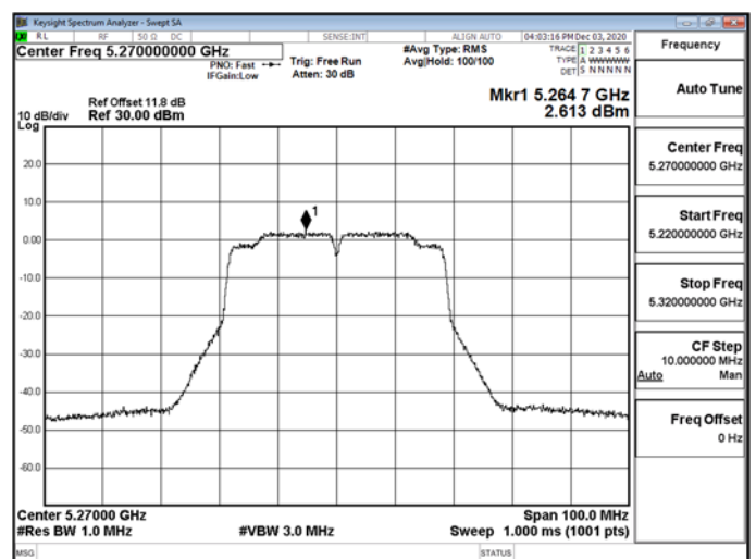
802.11n_40MHz_CH0_5270MHz-5270
