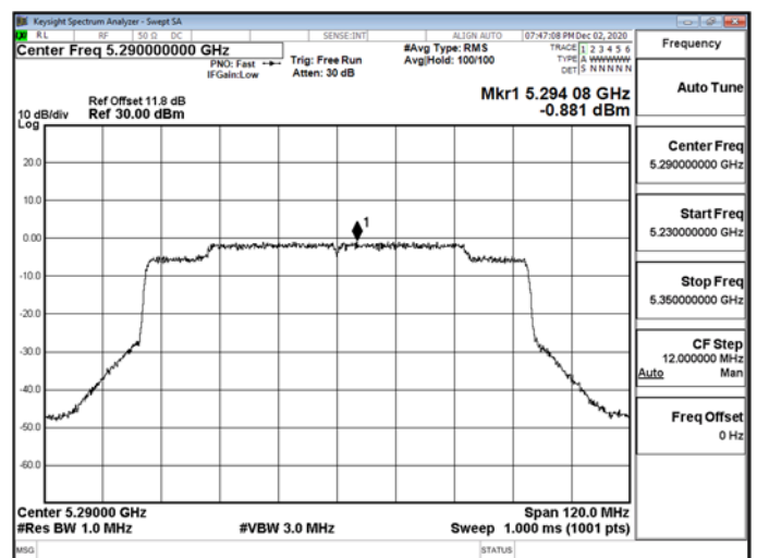
802.11ax_80MHz_5290MHz-5290
