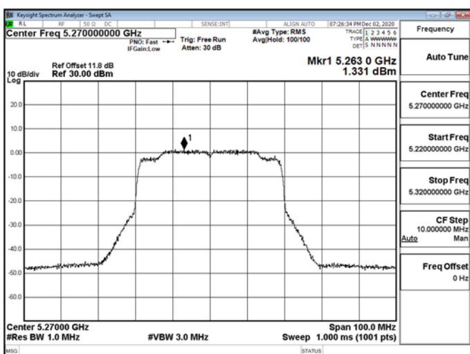
802.11ax_40MHz_5270MHz-5270
