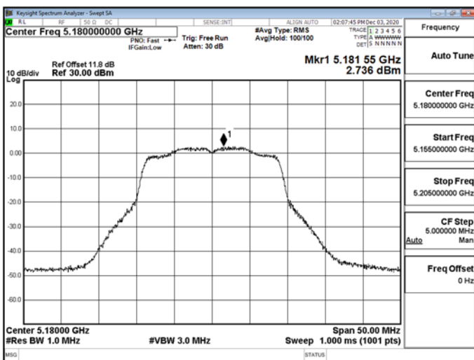
802.11n_20MHz_CH0_5180MHz-5180
