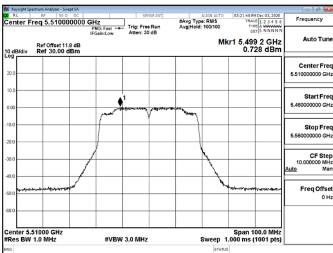
802.11n_40MHz_CH1_5510MHz-5510
