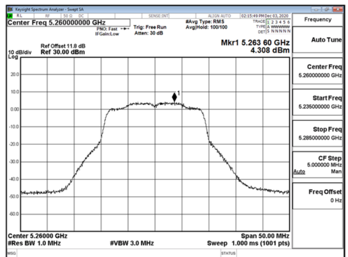
802.11n_20MHz_CH0_5260MHz-5260
