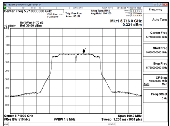
802.11n_40MHz_CHO_5710MHz_UNII 3
