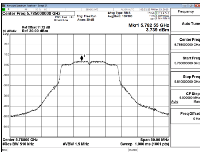
802.11n_20MHz_CHO_5785MHz-5785
