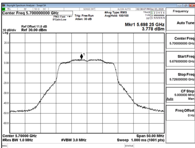
802.11n_20MHz_CH1_5700MHz-5700
