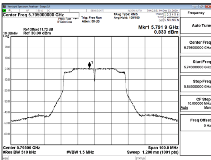
802.11n_40MHz_CH1_5795MHz-5795
