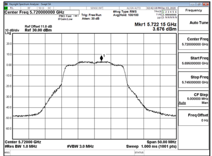
802.11n_20MHz_CH1_5720MHz_UNII 3
