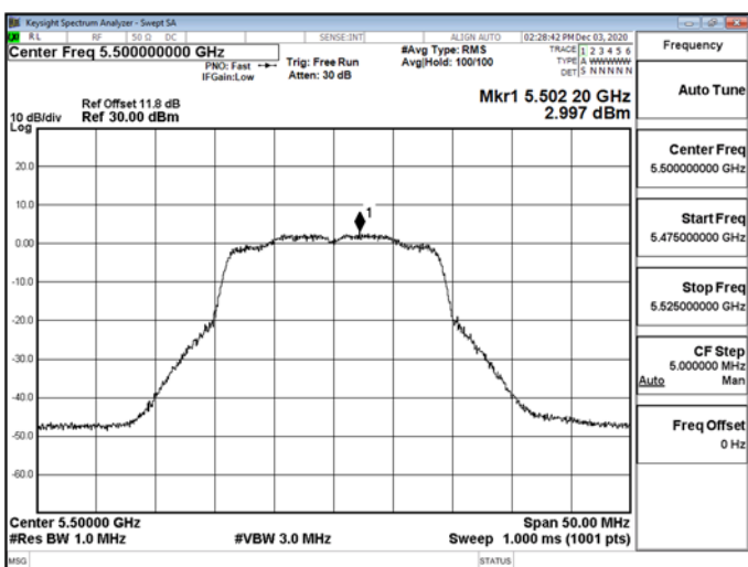
802.11n_20MHz_CHO_5500MHz-5500
