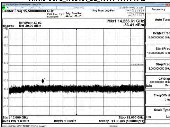
30MHz~3GHz_WCDMA_B2_13000-18000 MHz
