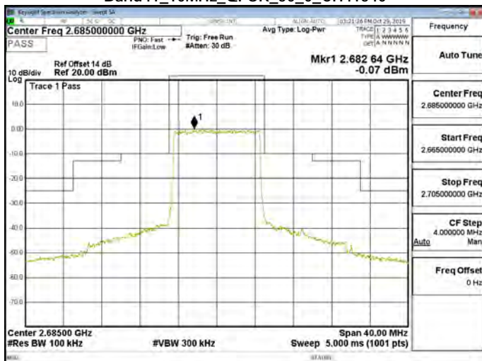
Band41_10MHz_QPSK_50_0_CH41540
