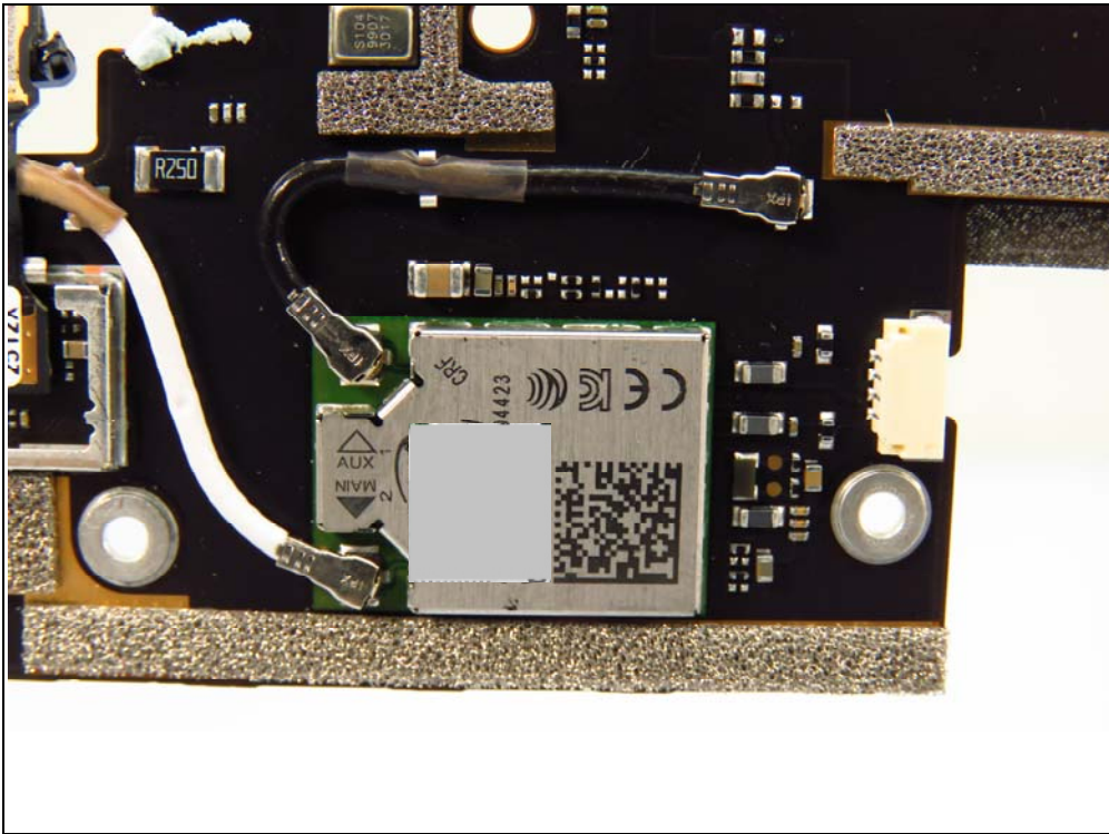
WiFi/BT module
