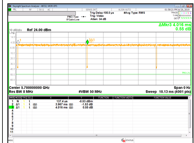
802.11ax HE20 OFDMA, SU MODE
