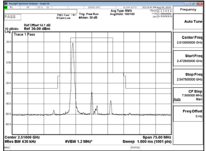
Band 7_20M_QPSK_LOW_RB1,99
