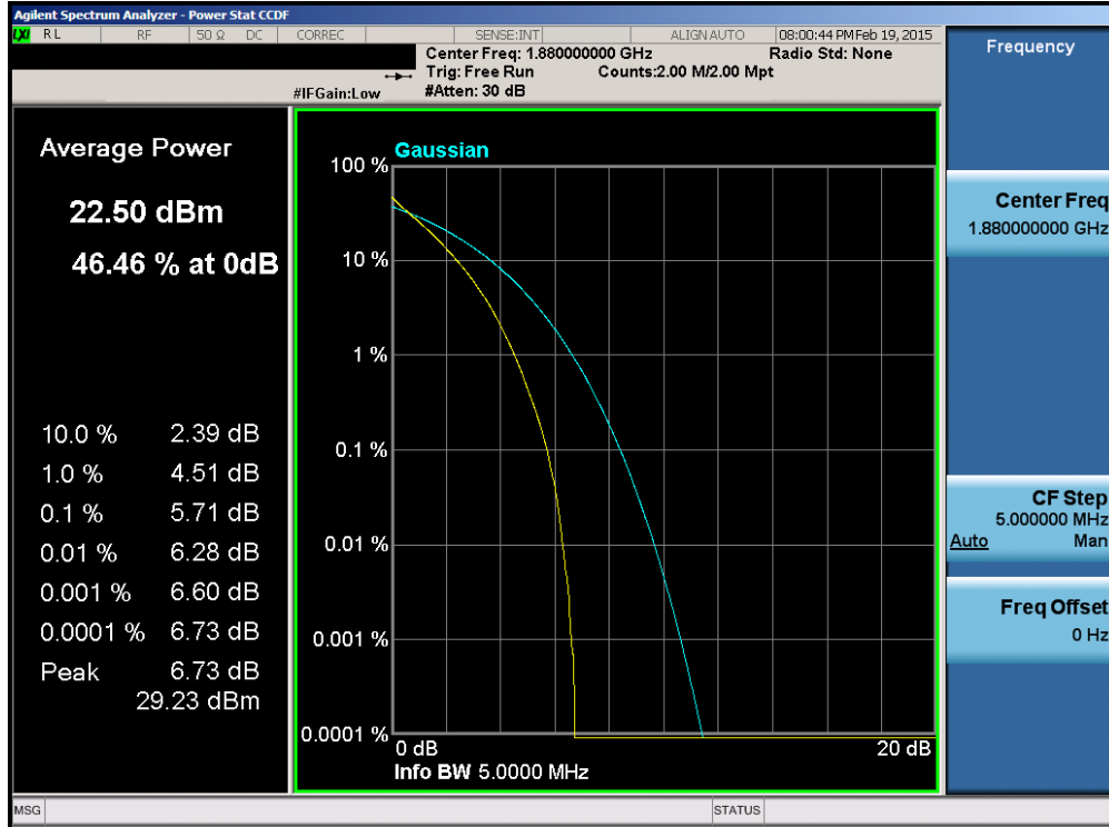
Plot 6-168. PAR Plot (Band 2 – 5.0MHz QPSK – RB Size 25)
