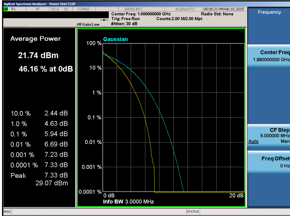
Plot 6-166. PAR Plot (Band 2 – 3.0MHz QPSK – RB Size 15)
