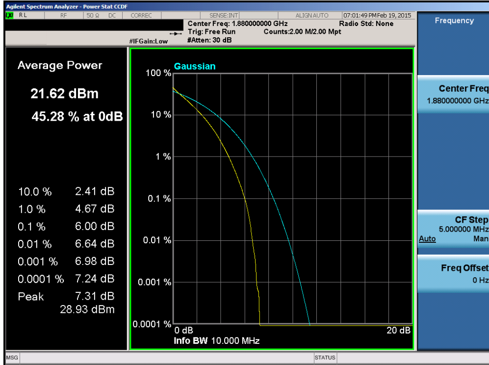
Plot 6-170. PAR Plot (Band 2 – 10.0MHz QPSK – RB Size 50)
