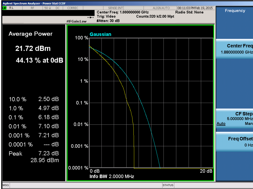
Plot 6-164. PAR Plot (Band 2 – 1.4MHz QPSK – RB Size 6)
