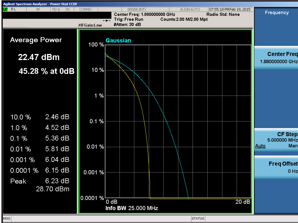
Plot 6-174. PAR Plot (Band 2 – 20.0MHz QPSK – RB Size 100)
