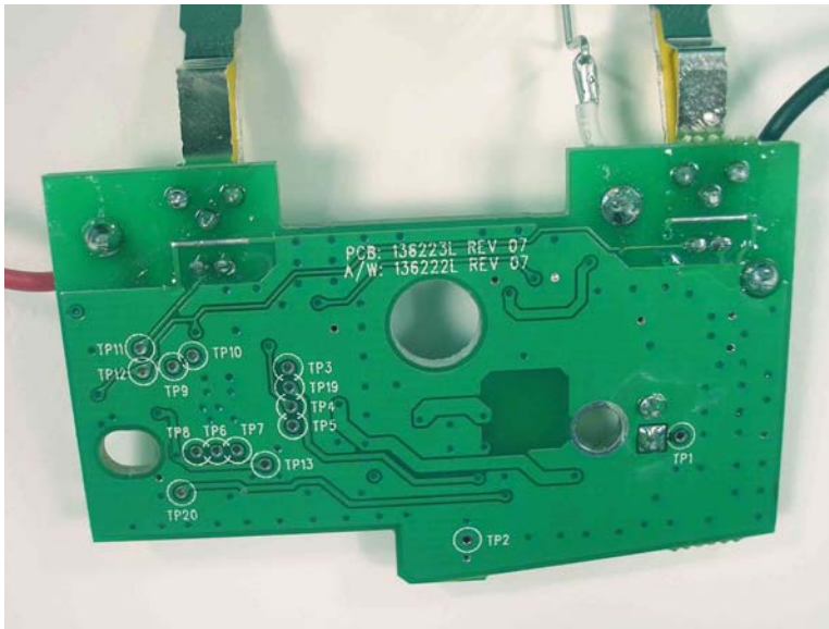
PCB 136223L Bottom
