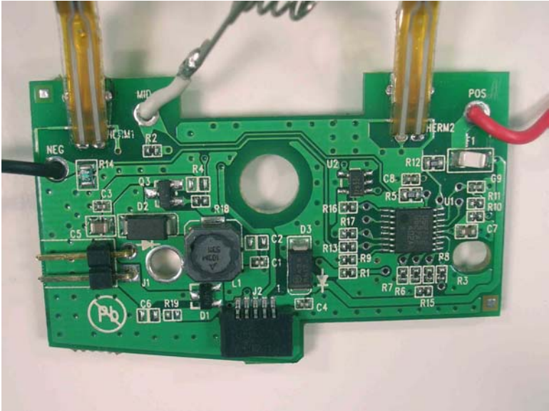
PCB 136223L Top
