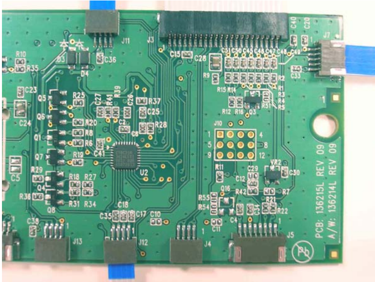
PCB 136215L Top Right
