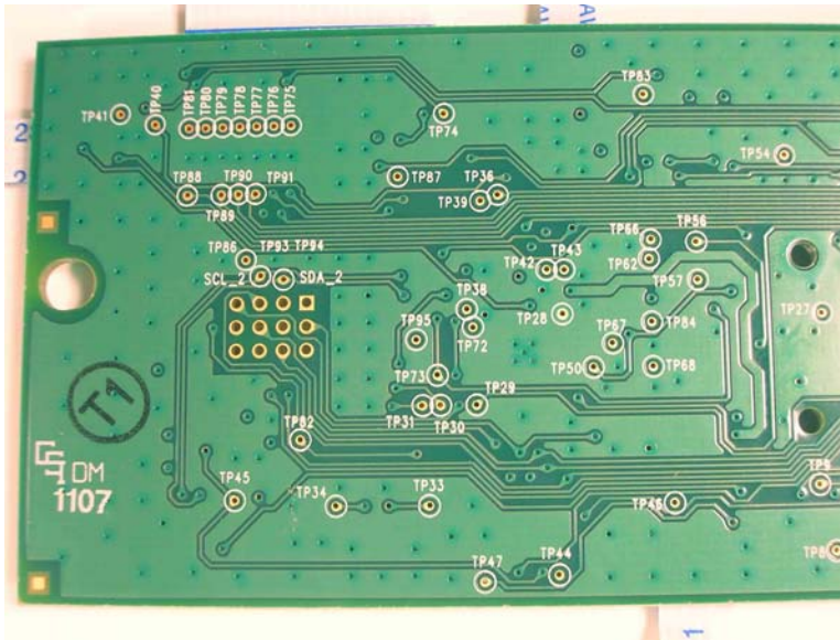
PCB 136215L Bottom Left
