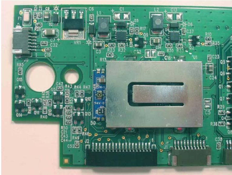
PCB 136215L Top Left
