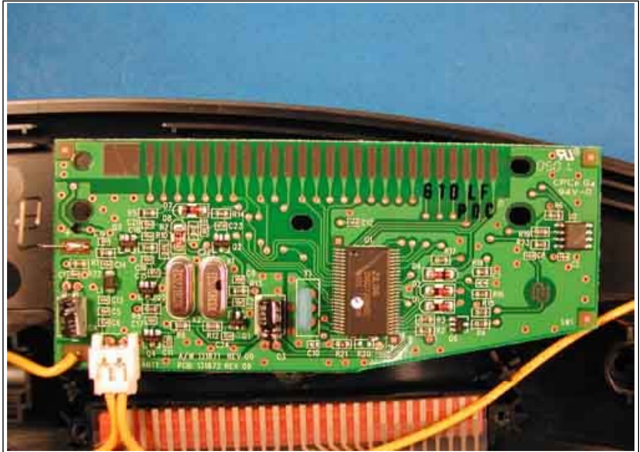
PCB Bottom
