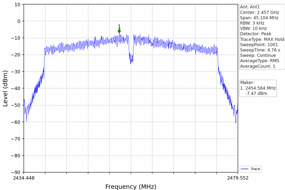
11N40_MCH_2457MHz_Ant1_NTNV
