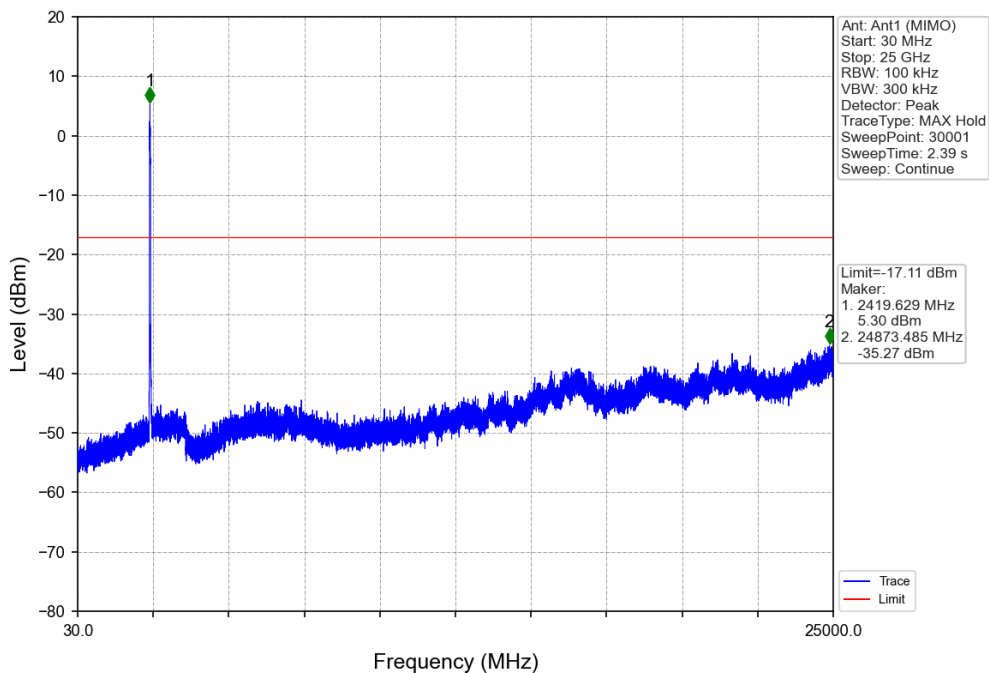
802.11n(HT40)_LCH_2422MHz_Ant1 (MIMO)_NTNV
