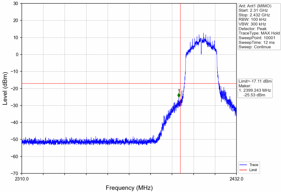
802.11n(HT20)_LCH_2412MHz_Ant1 (MIMO)_NTNV
