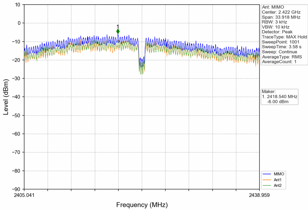
802.11n(HT40)_LCH_2422MHz_MIMO_NTNV
