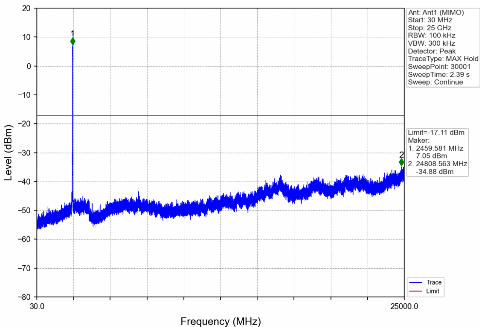
802.11n(HT20)_HCH_2462MHz_Ant1 (MIMO)_NTNV
