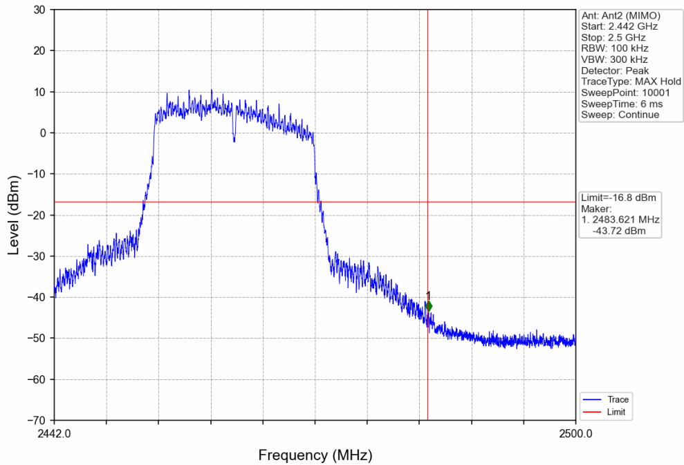
802.11n(HT20)_HCH_2462MHz_Ant2 (MIMO)_NTNV
