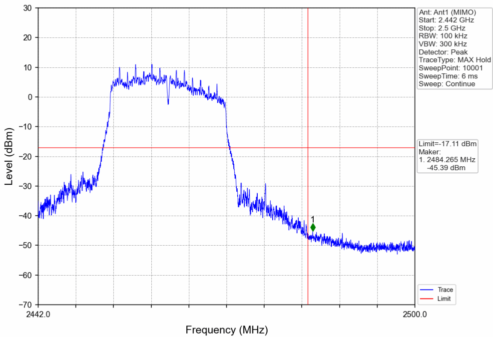
802.11n(HT20)_HCH_2462MHz_Ant1 (MIMO)_NTNV
