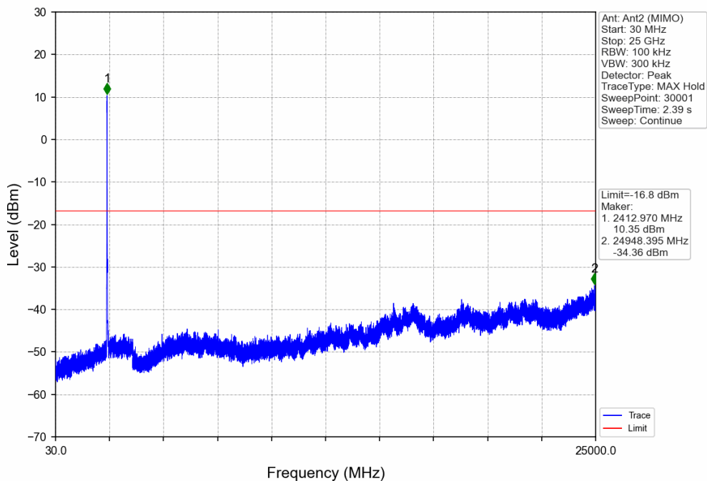
802.11n(HT20)_LCH_2412MHz_Ant2 (MIMO)_NTNV
