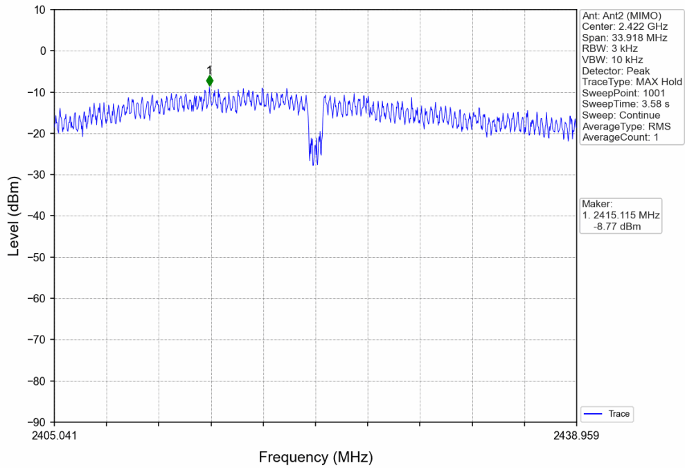
802.11n(HT40)_LCH_2422MHz_MIMO_NTNV
