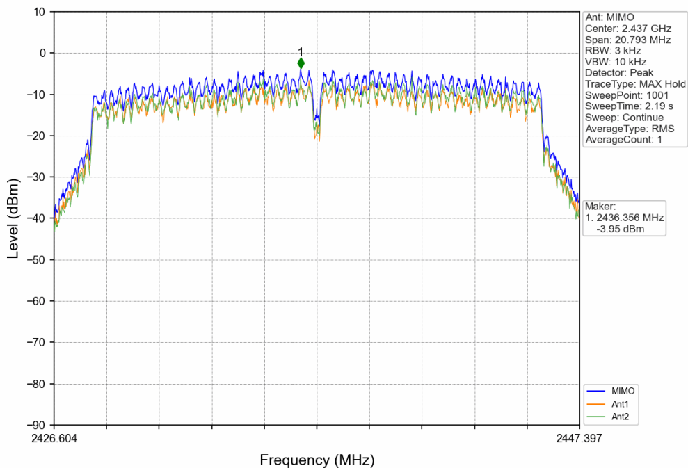
802.11n(HT20)_MCH_2437MHz_MIMO_NTNV
