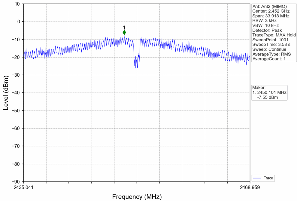
802.11n(HT40)_HCH_2452MHz_MIMO_NTNV
