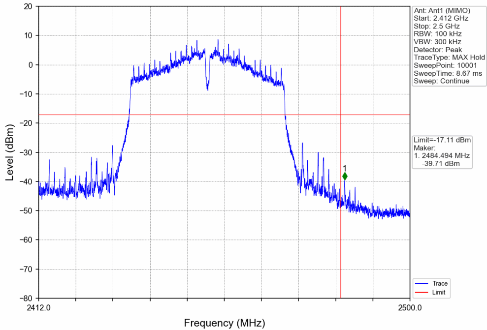
802.11n(HT40)_HCH_2452MHz_Ant1 (MIMO)_NTNV
