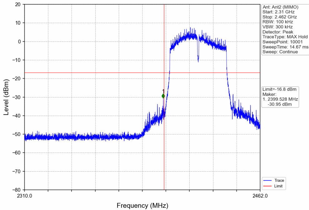
802.11n(HT40)_LCH_2422MHz_Ant2 (MIMO)_NTNV
