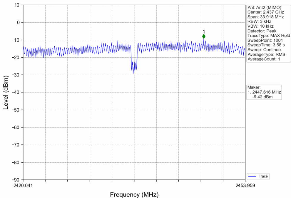
802.11n(HT40)_MCH_2437MHz_Ant2 (MIMO)_NTNV
