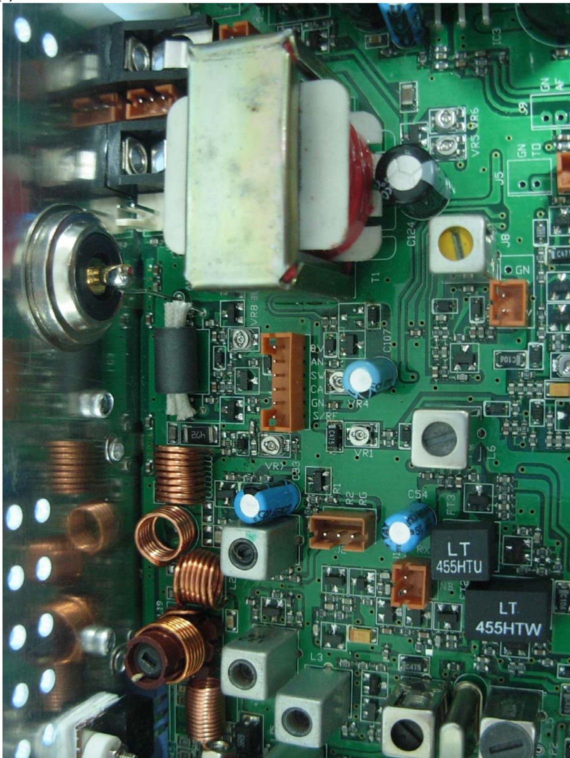
(9) EUT Photo
