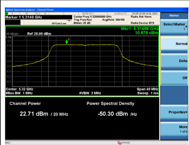
5320MHz-PWR
