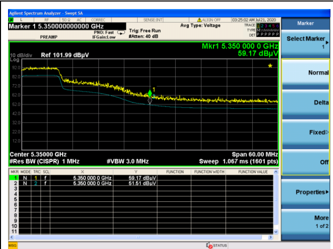
5320MHz- Edge 5350MHz
