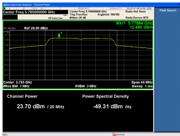
5785MHz-PWR
