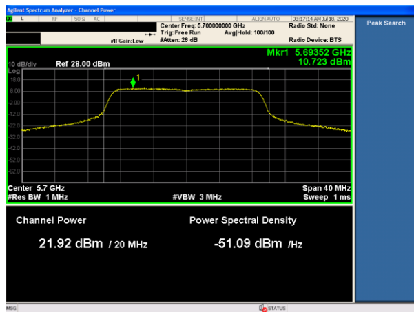
5700MHz-PWR
