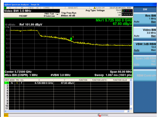
5700MHz- Edge 5725MHz
