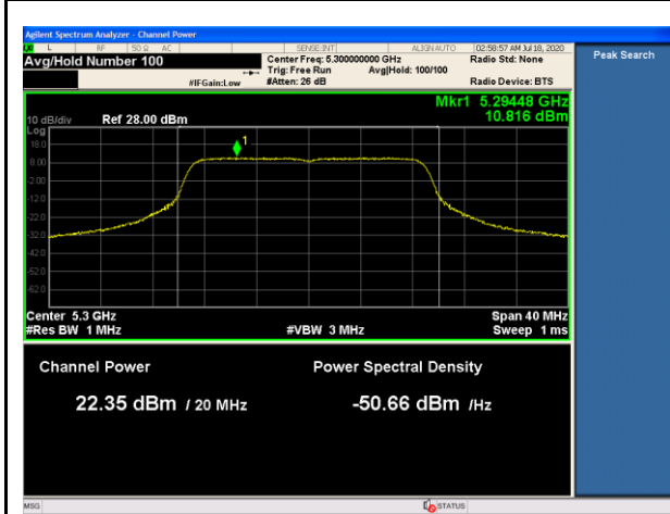
5300MHz-PWR
