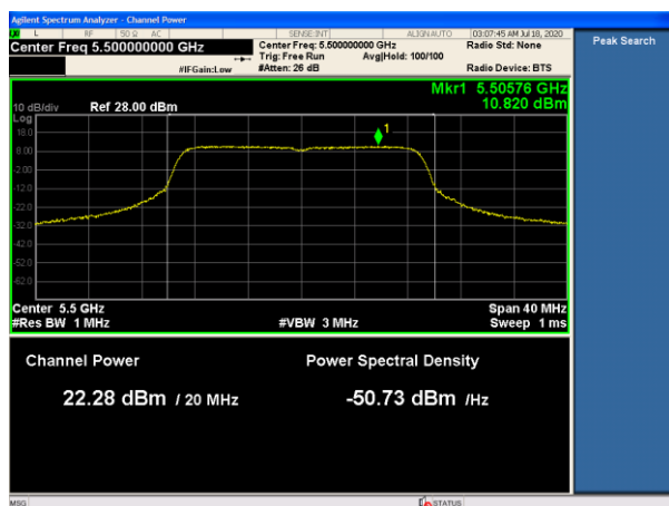
5500MHz-PWR
