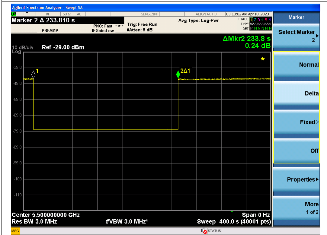
Initial CAC -5500MHz
