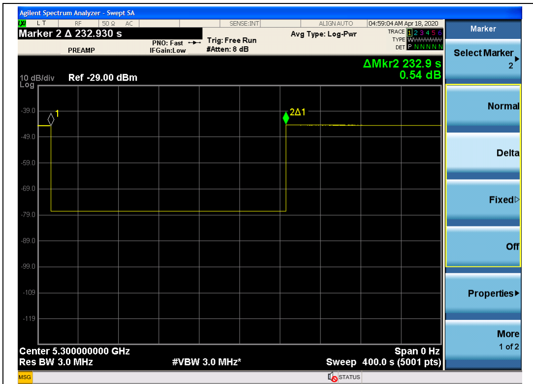
Initial CAC -5300MHz
