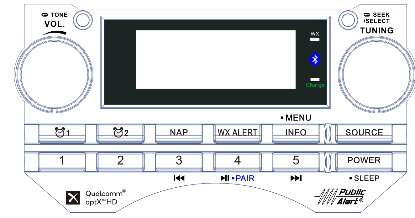
面版正視
