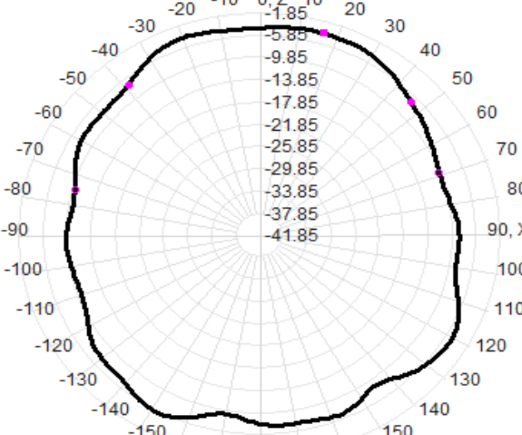
2470.0MHz Total(E1-XZ), Max=-3.82dBi
