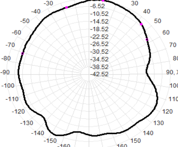
2400.0MHz Total(E1-XZ), Max=-2.65dBi
