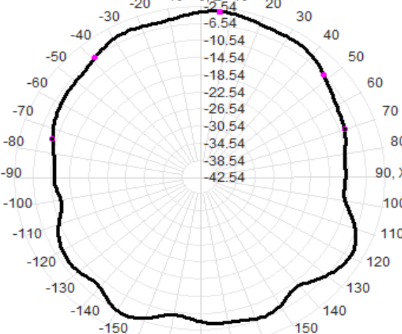
2450.0MHz Total(E1-XZ), Max=-3.97dBi
