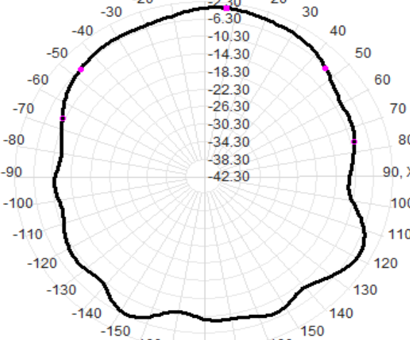
2430.0MHz Total(E1-XZ), Max=-3.56dBi
