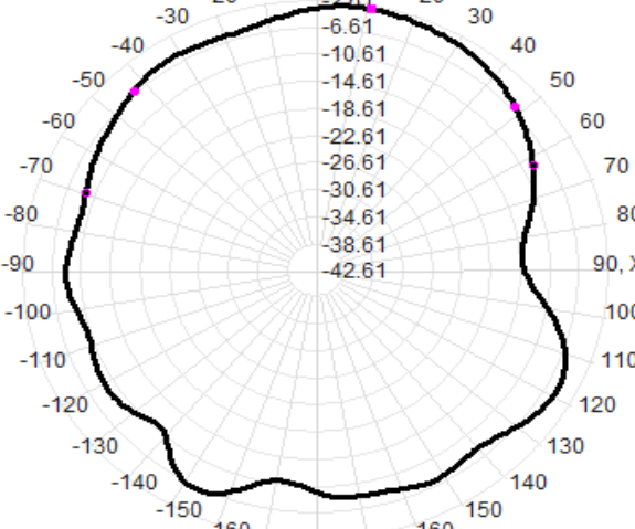
2420.0MHz Total(E1-XZ), Max=-3.23dBi
