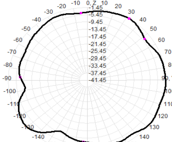
2500.0MHz Total(E2-YZ), Max=-0.70dBi
