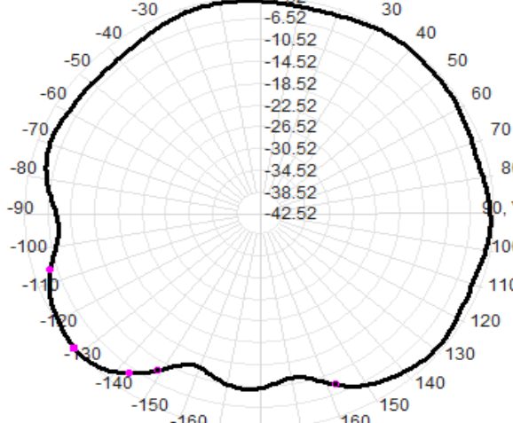
2400.0MHz Total(E2-YZ), Max=-2.52dBi
