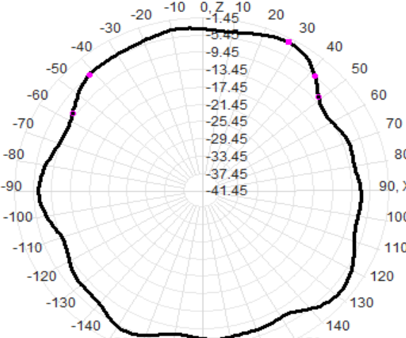
2500.0MHz Total(E1-XZ), Max=-2.18dBi
