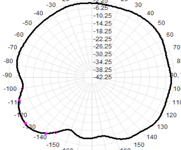
2430.0MHz Total(E2-YZ), Max=-2.30dBi
