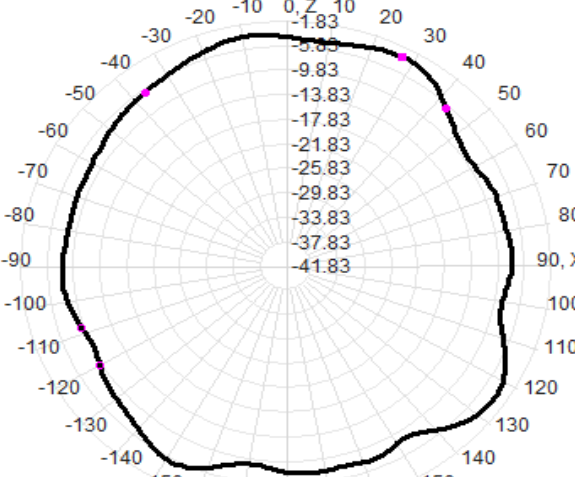
2480.0MHz Total(E1-XZ), Max=-3.45dBi
