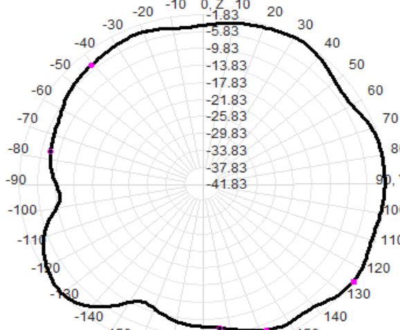
2480.0MHz Total(E2-YZ), Max=-1.83dBi
