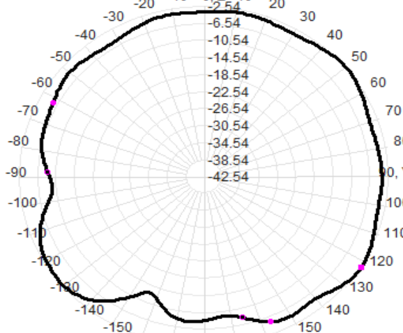
2450.0MHz Total(E2-YZ), Max=-2.08dBi
