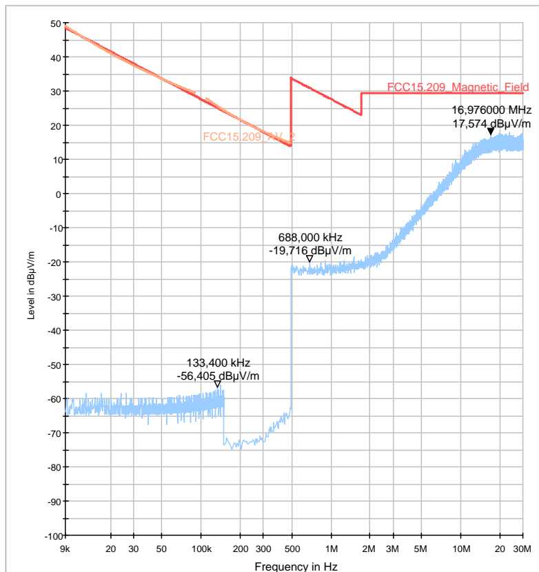
FCC15.209_magn hor+vert
