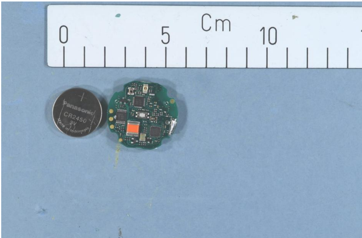
NITX – PCB Front side
