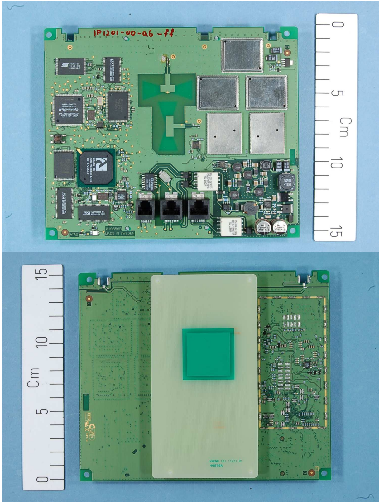
ASCOM IPBS1
