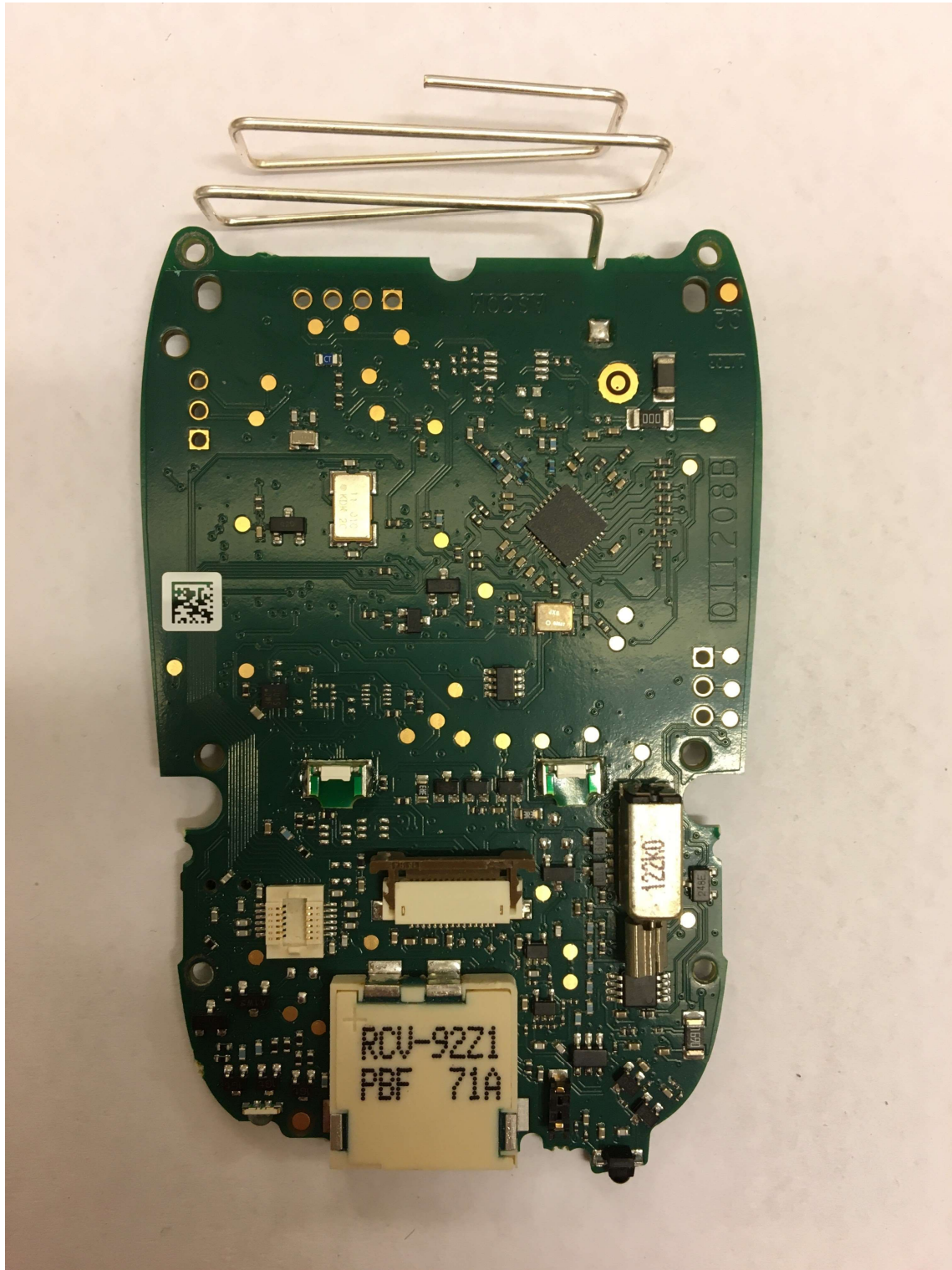
PCB top side:
