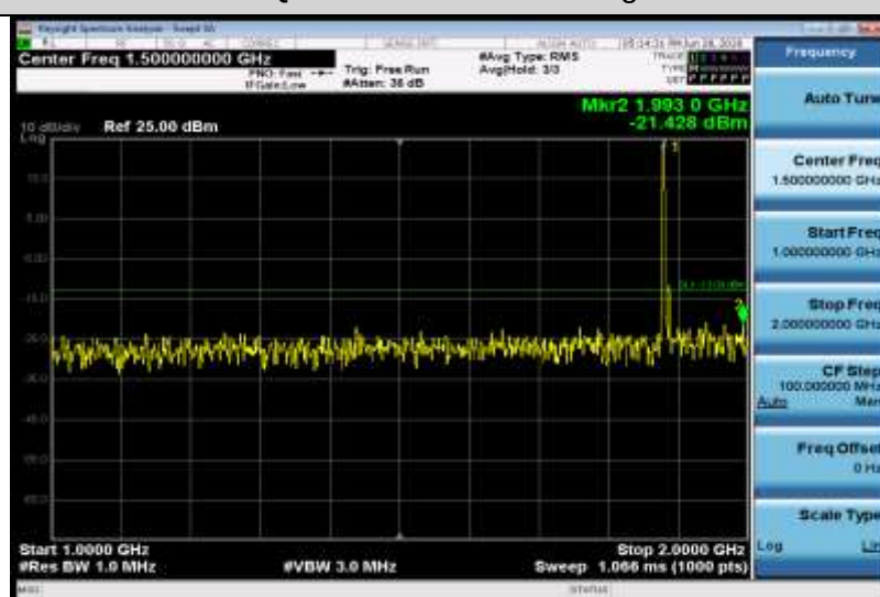
Band25-10MHz-16QAM-26365-1RB#0-Range2:1000~2000MHz
