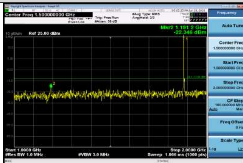
Band25-5MHz-QPSK-26365-1RB#0-Range2:1000~2000MHz
