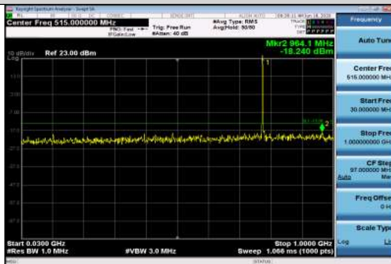
Band13-5MHz-QPSK-23230-1RB#0-Range1:30~1000MHz
