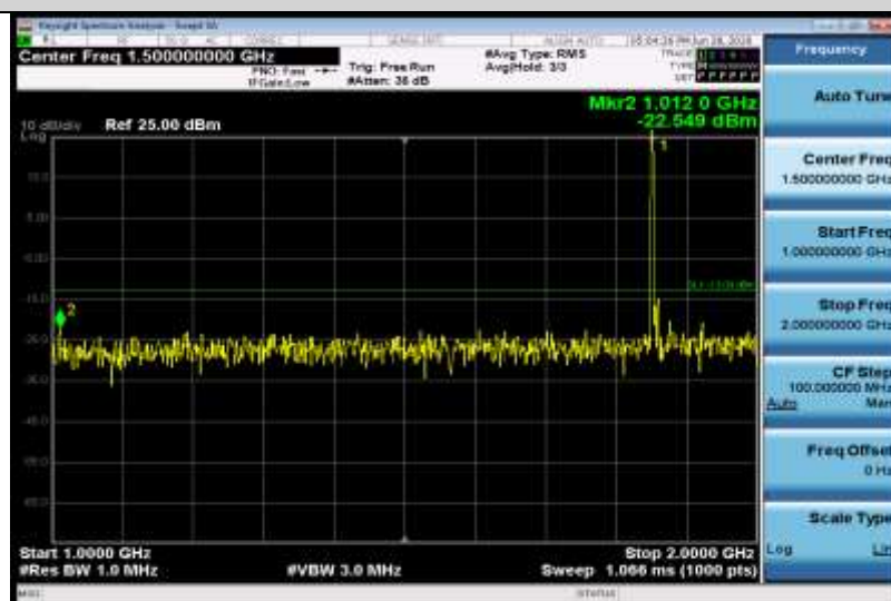
Band25-5MHz-QPSK-26065-1RB#0-Range2:1000~2000MHz
