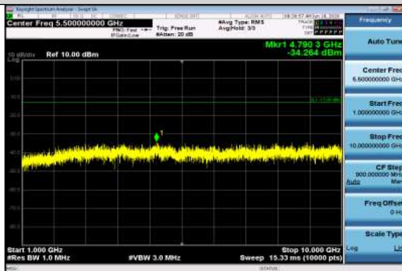
Band12-3MHz-QPSK-23165-1RB#0-Range2:1000~10000MHz
