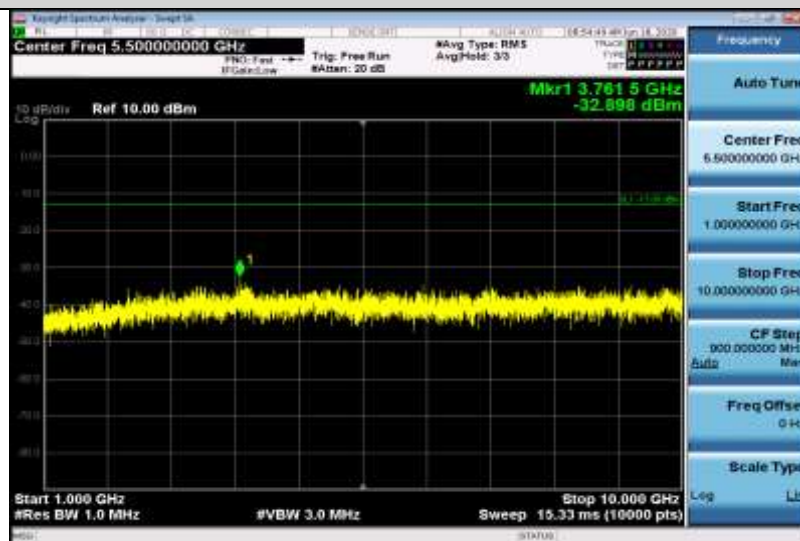
Band12-5MHz-QPSK-23155-1RB#0-Range2:1000~10000MHz
