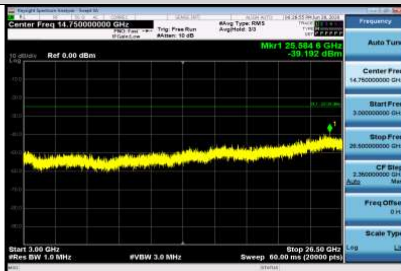
Band7-5MHz-QPSK-21425-1RB#0-Range3:3000~26500MHz
