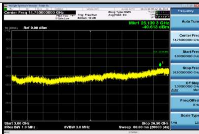
Band7-10MHz-QPSK-20800-1RB#0-Range3:3000~26500MHz
