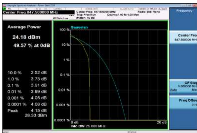
Band5-3MHz-QPSK-20635-15RB#0
