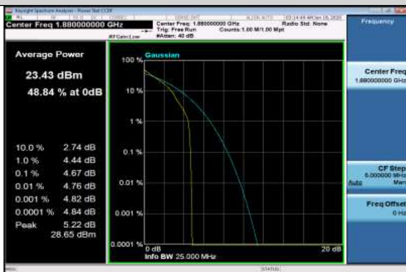
Band2-10MHz-QPSK-18900-50RB#0
