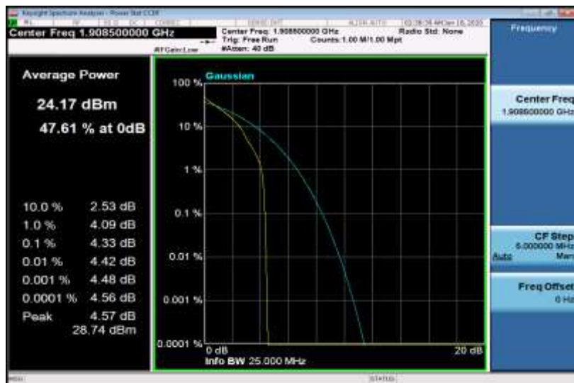
Band2-3MHz-QPSK-19185-15RB#0
