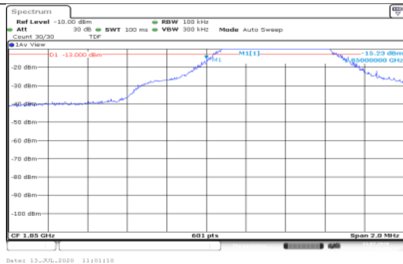
Band2-5MHz-QPSK-18625-1RB#24
