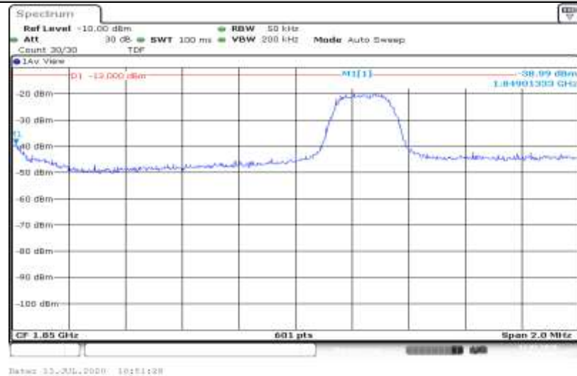
Band2-3MHz-16QAM-18615-15RB#0
