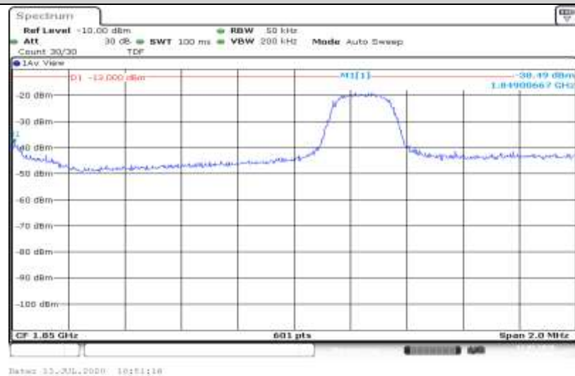
Band2-3MHz-QPSK-18615-1RB#14
