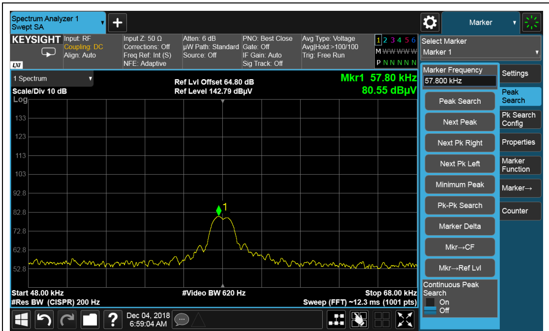
Fundamental – 58kHz
