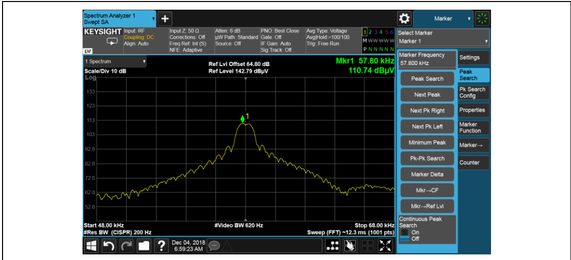
Fundamental – 58kHz
