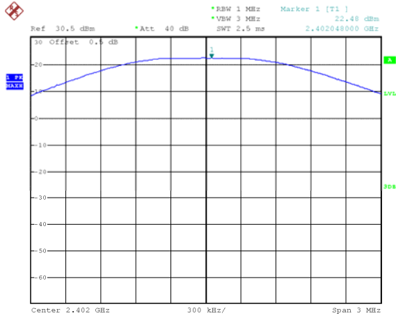
2.4G(ANT 1): channel 0
