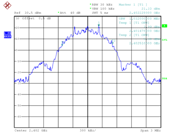
2.4G(ANT 1): channel 0
