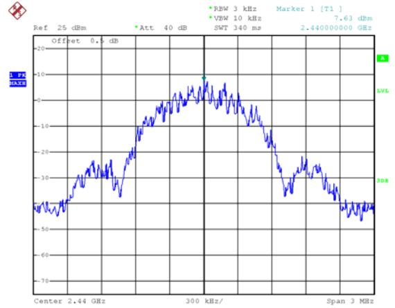
2.4G(ANT 1): channel 12
