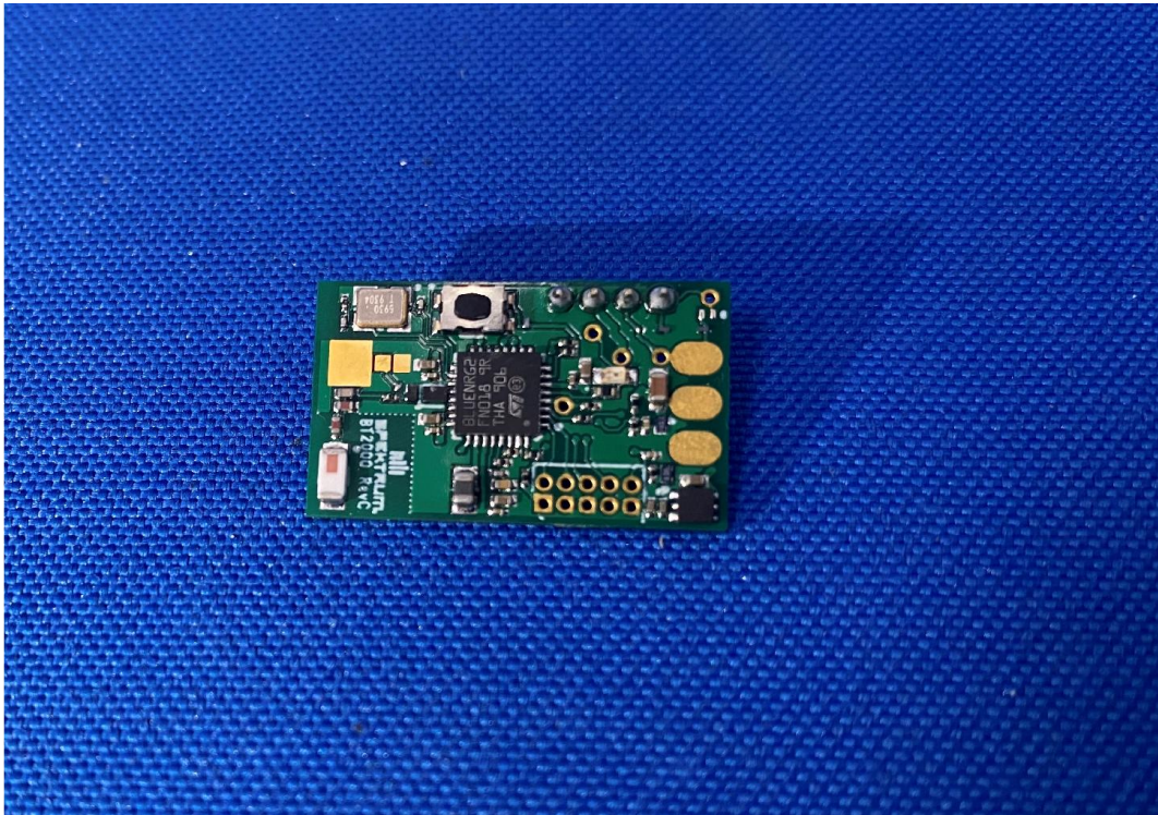
(3) EUT Photo
