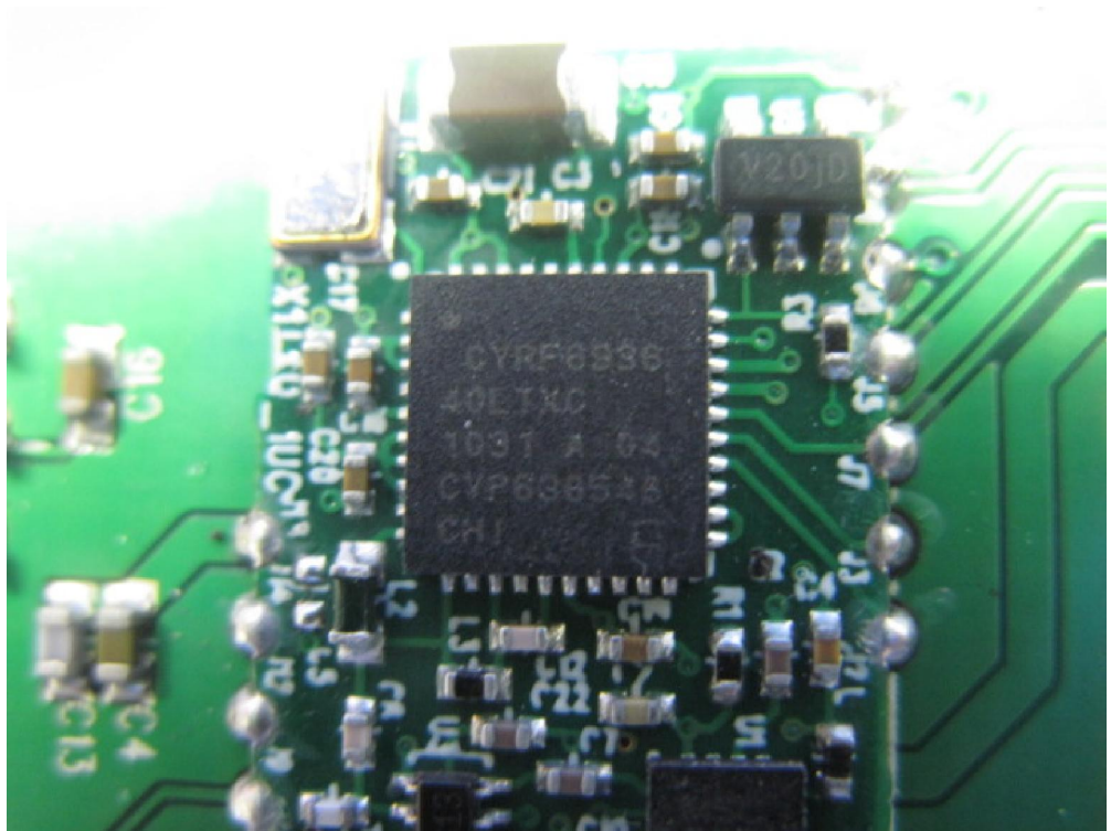
(5) EUT Photo
