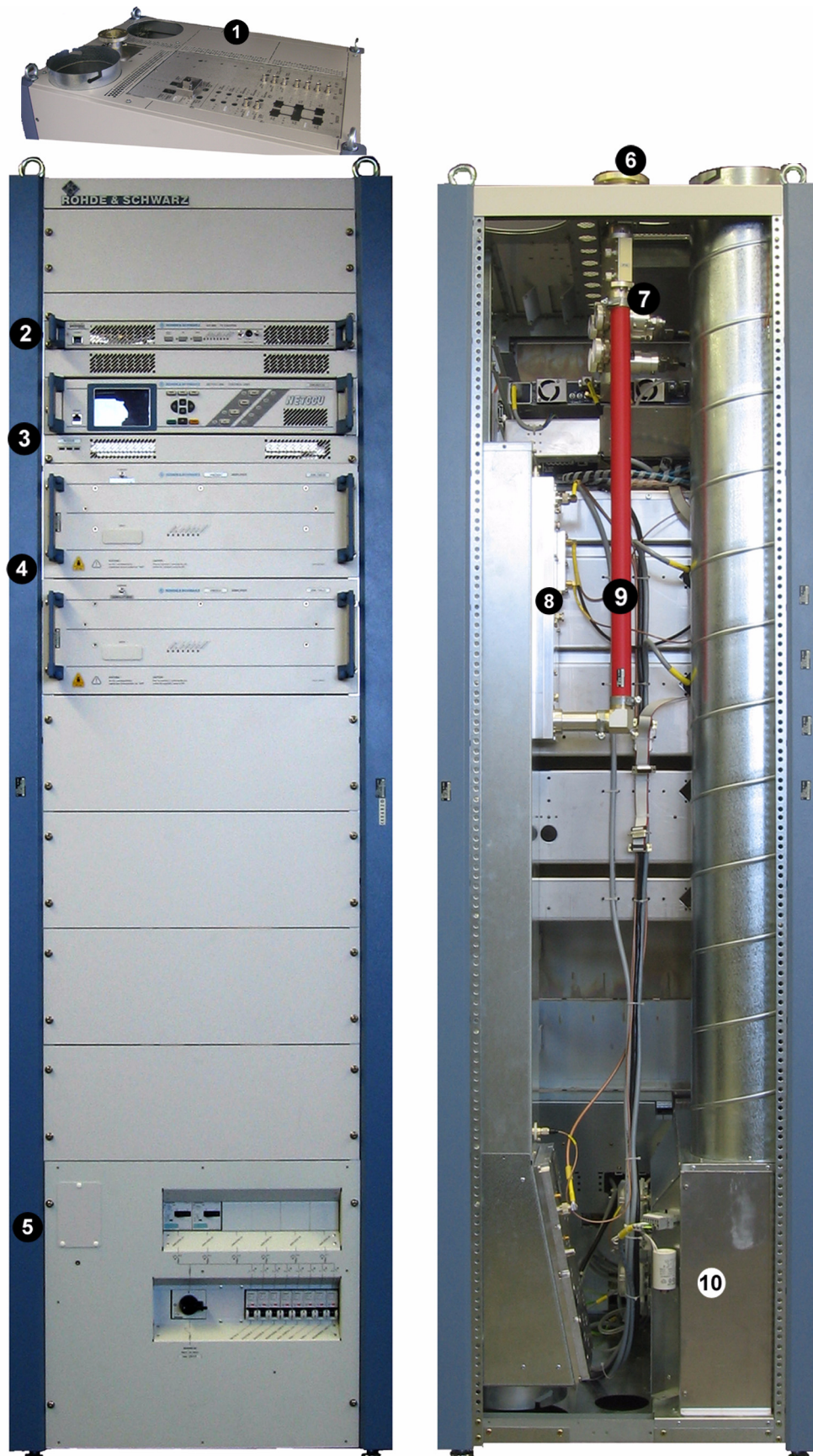
Fig. 2 Transmitter NW8202 modules
