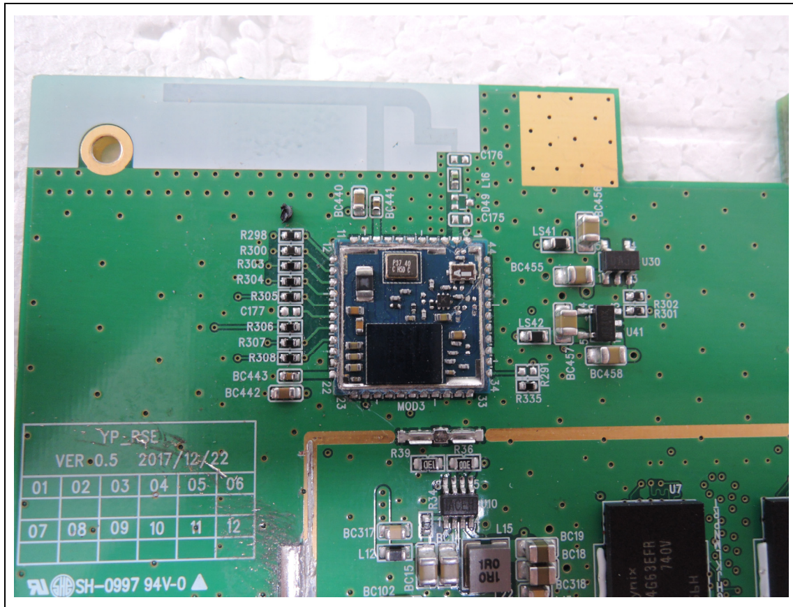
<WiFi Module>
