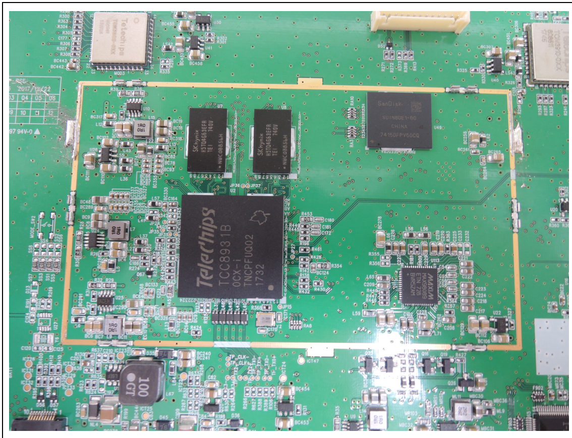
<Mainboard Module>
