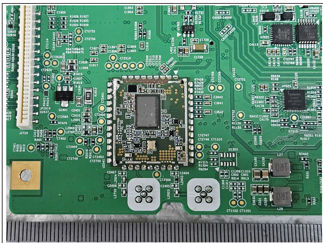
<BT/WLAN Module>
