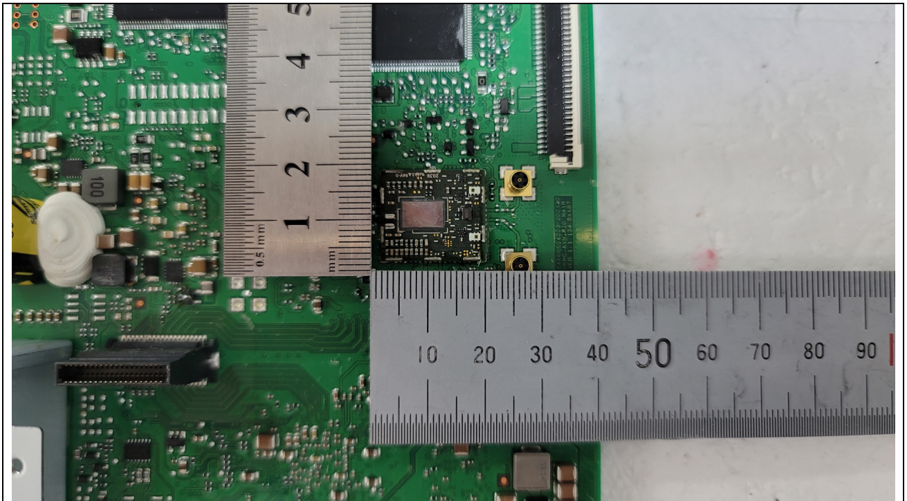
<Module>
