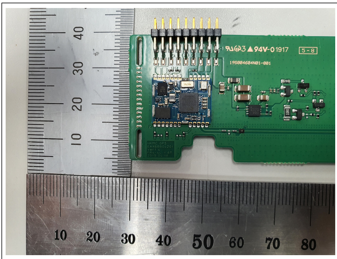
<GPS Module>
