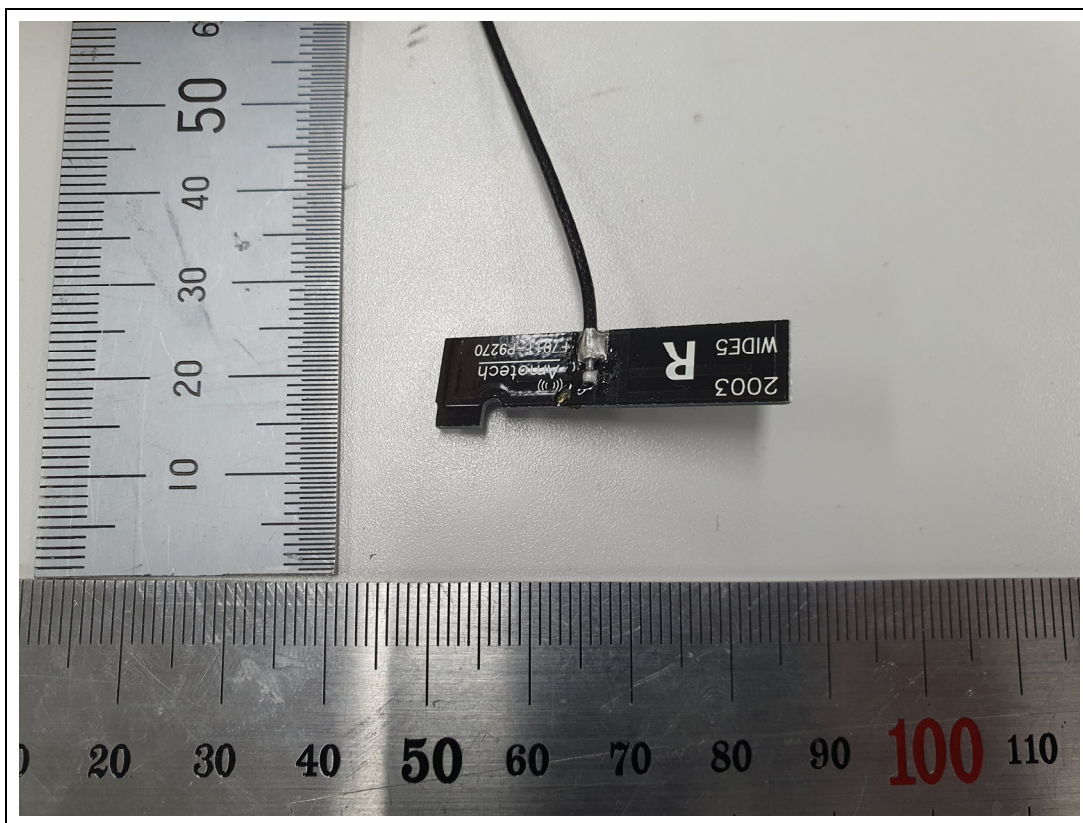
<Antenna 2>
