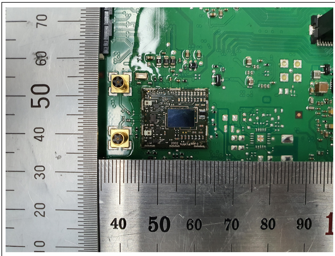
<BT,WiFi Module>
