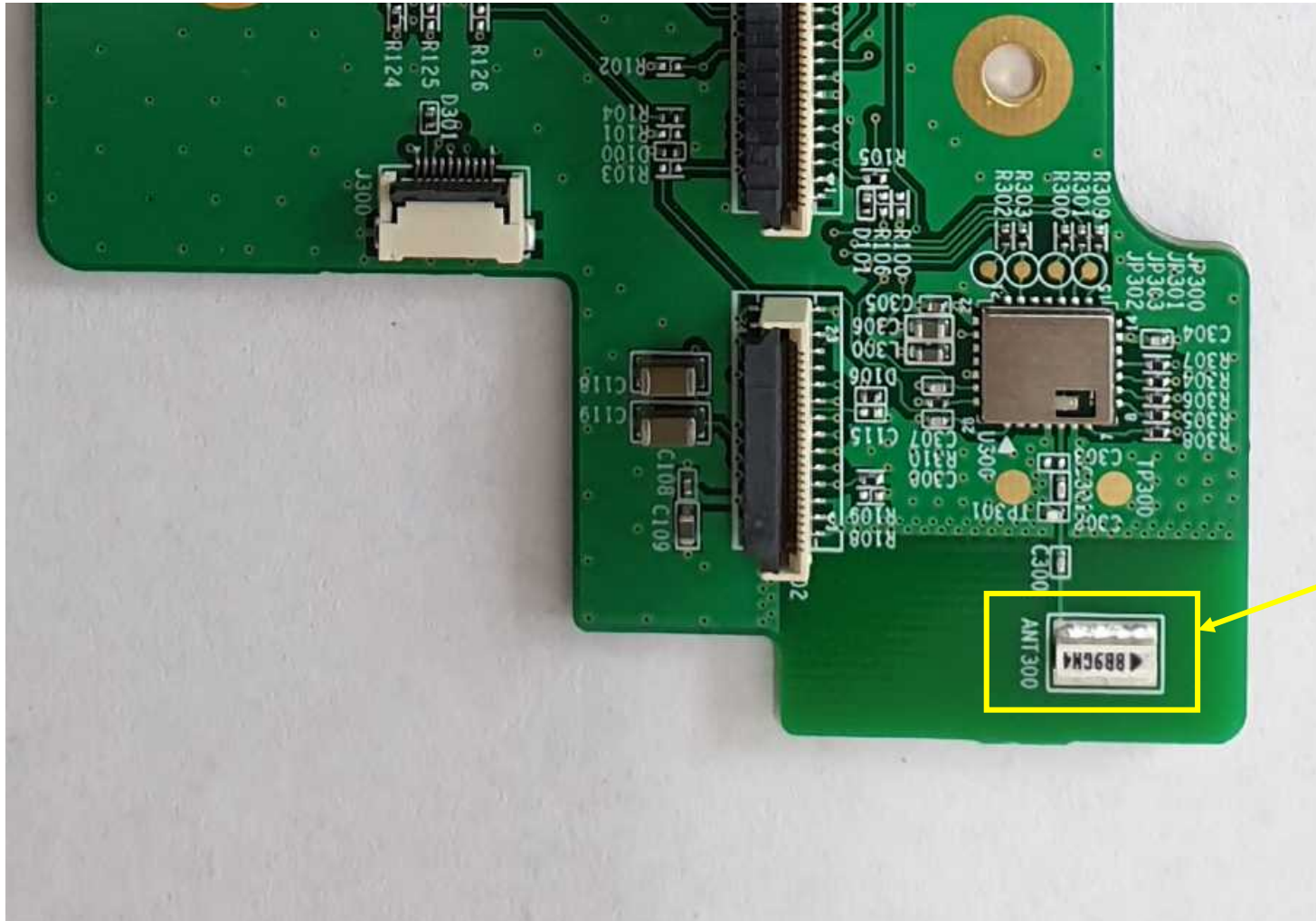
[Antenna]
