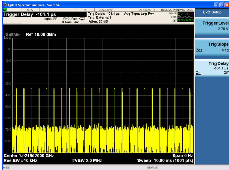
35 µs Pulses
