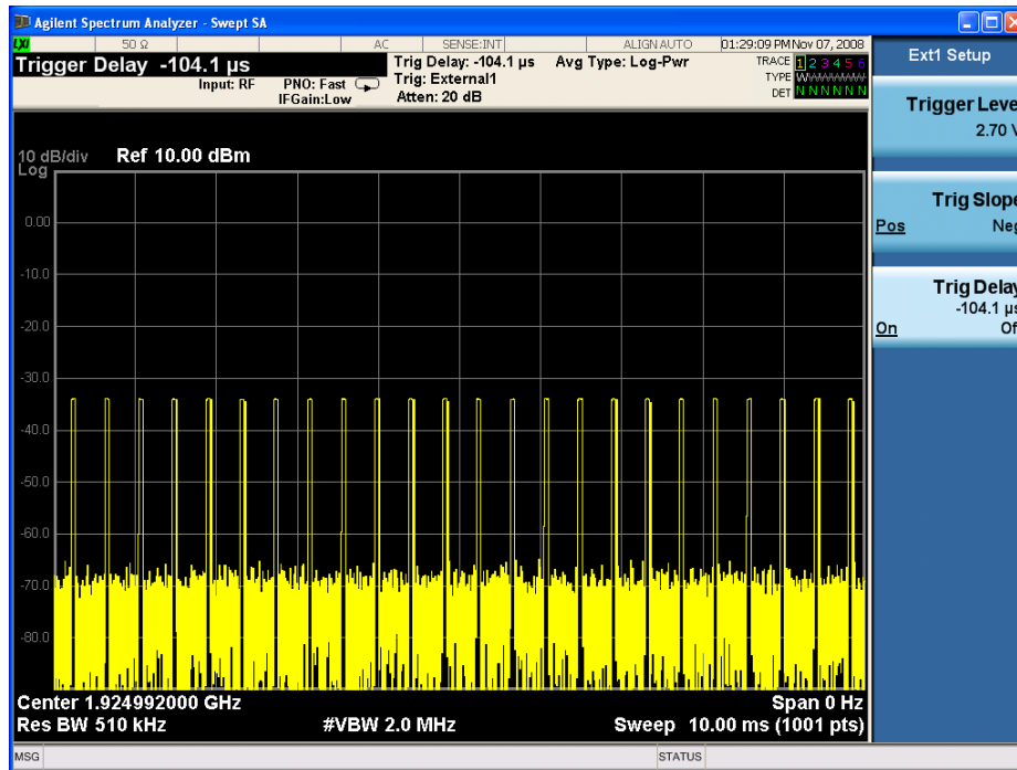
50 µs Pulses
