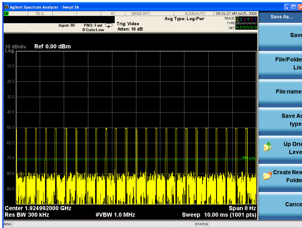
50 µs Pulses
